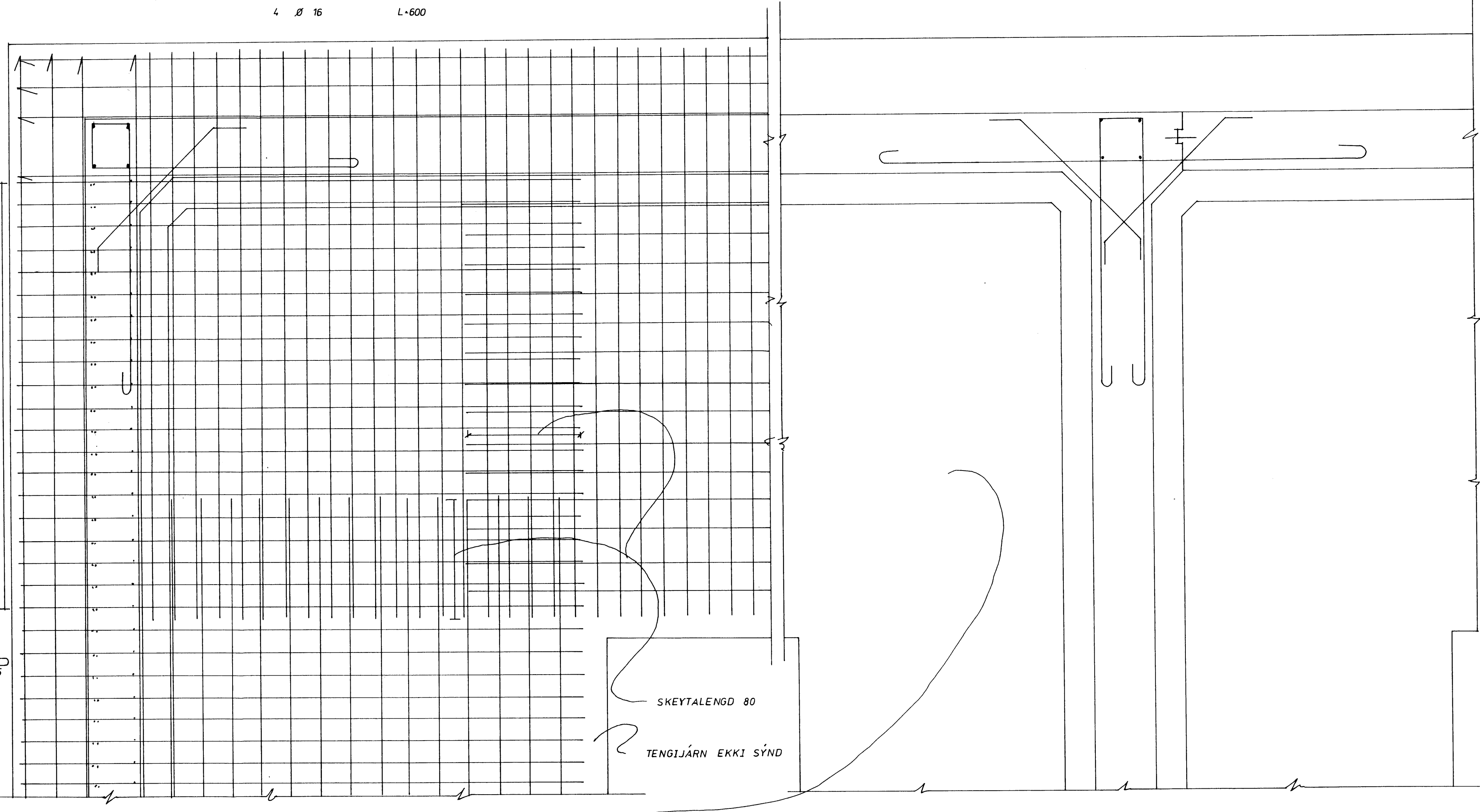
LÁRÉTT SNID Í HORN 1:20
