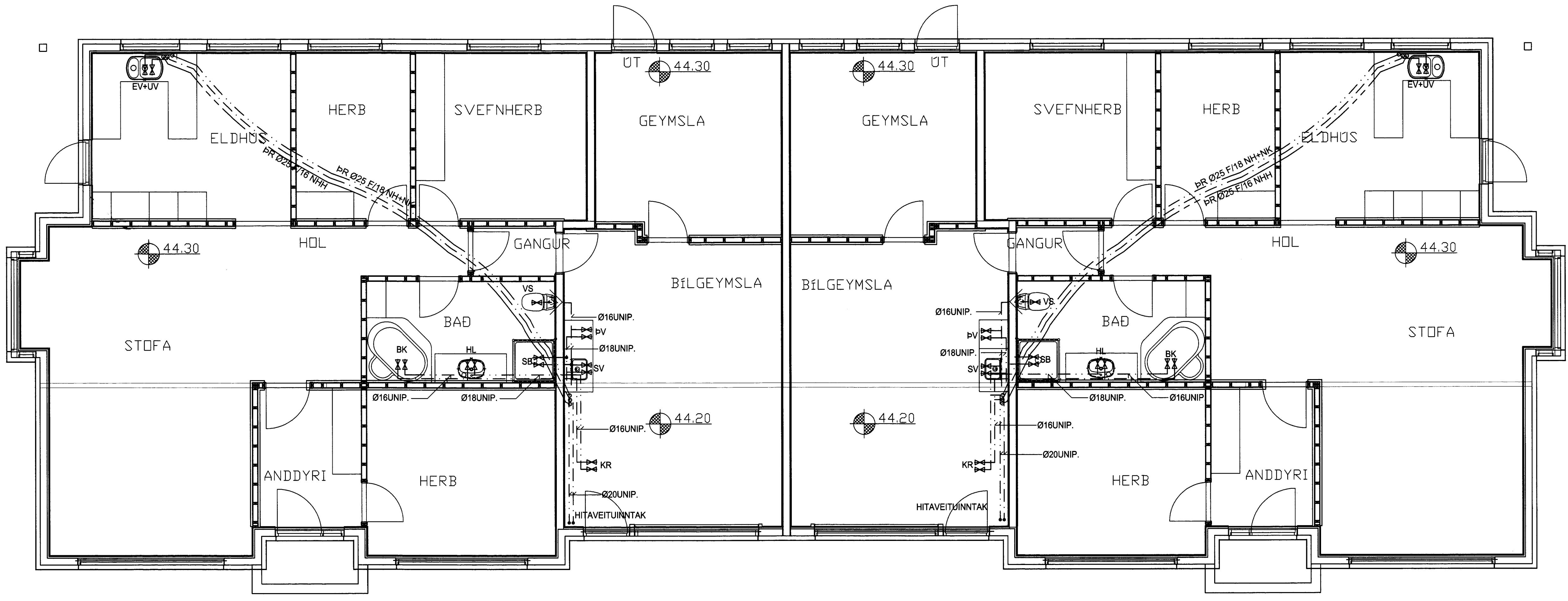
GRUNNMYND VATNSLAGNIR
