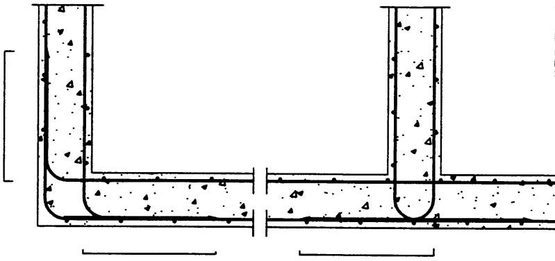
LAGNING LARÉTTA JÄRNA UM HÖRN Í VEGGJUM M=1:10
