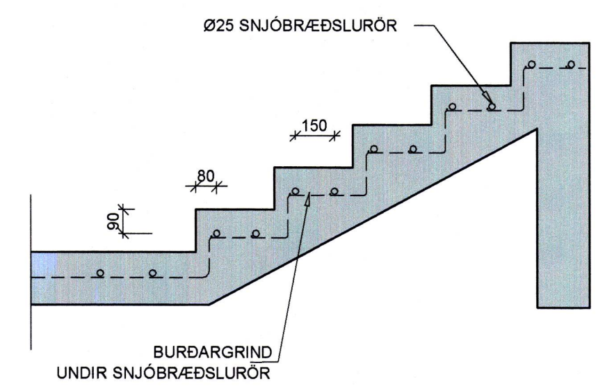
SNID Í SNJÓBRÆDSLULÖGN Í TRÖPPUM, 1:20
