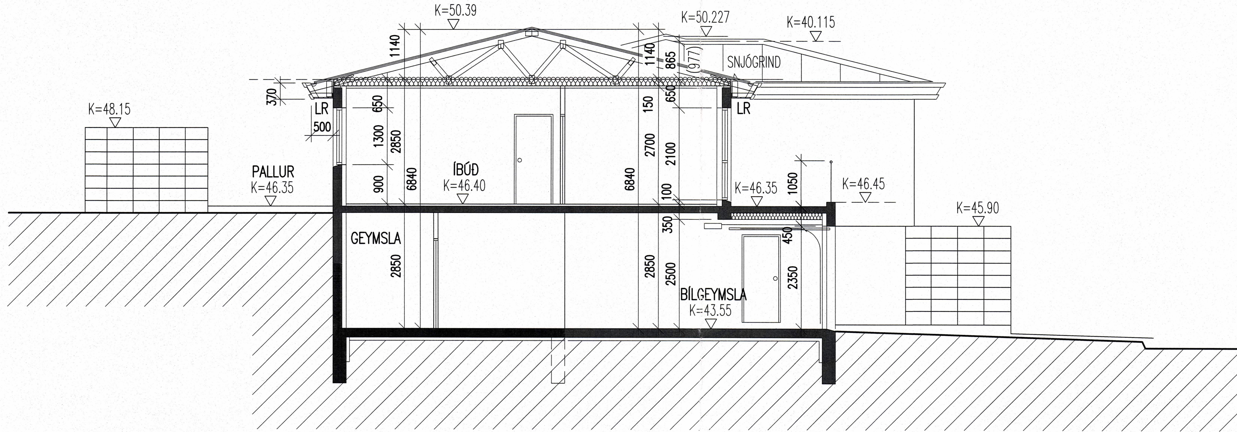
SNID-AA, MKV. 1:100
