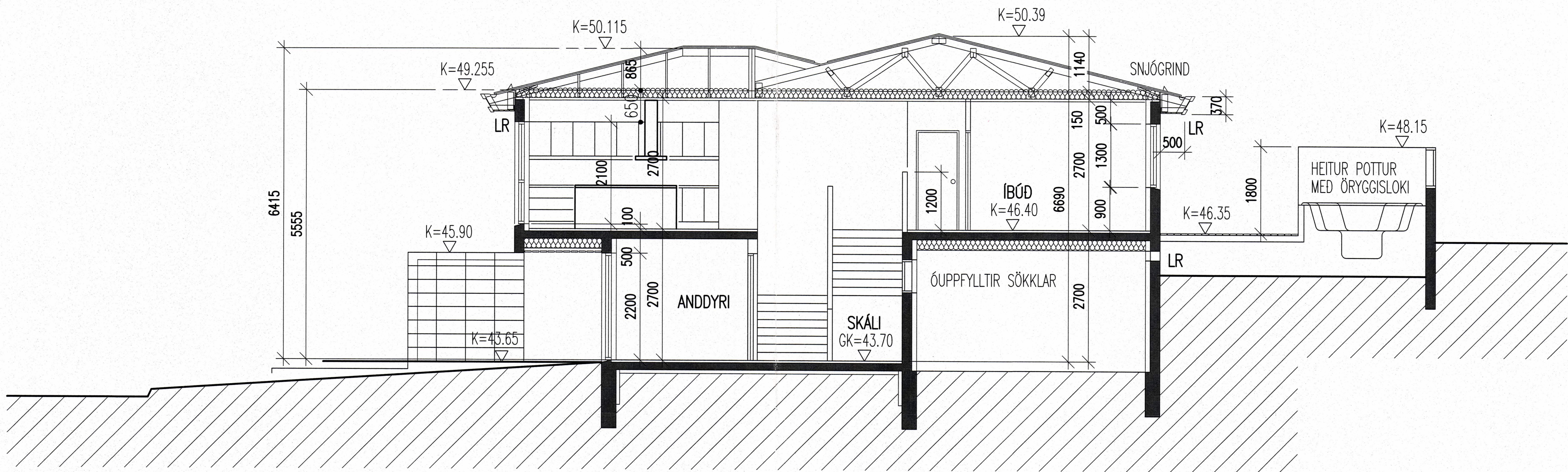
SNID-BB, MKV. 1:100
