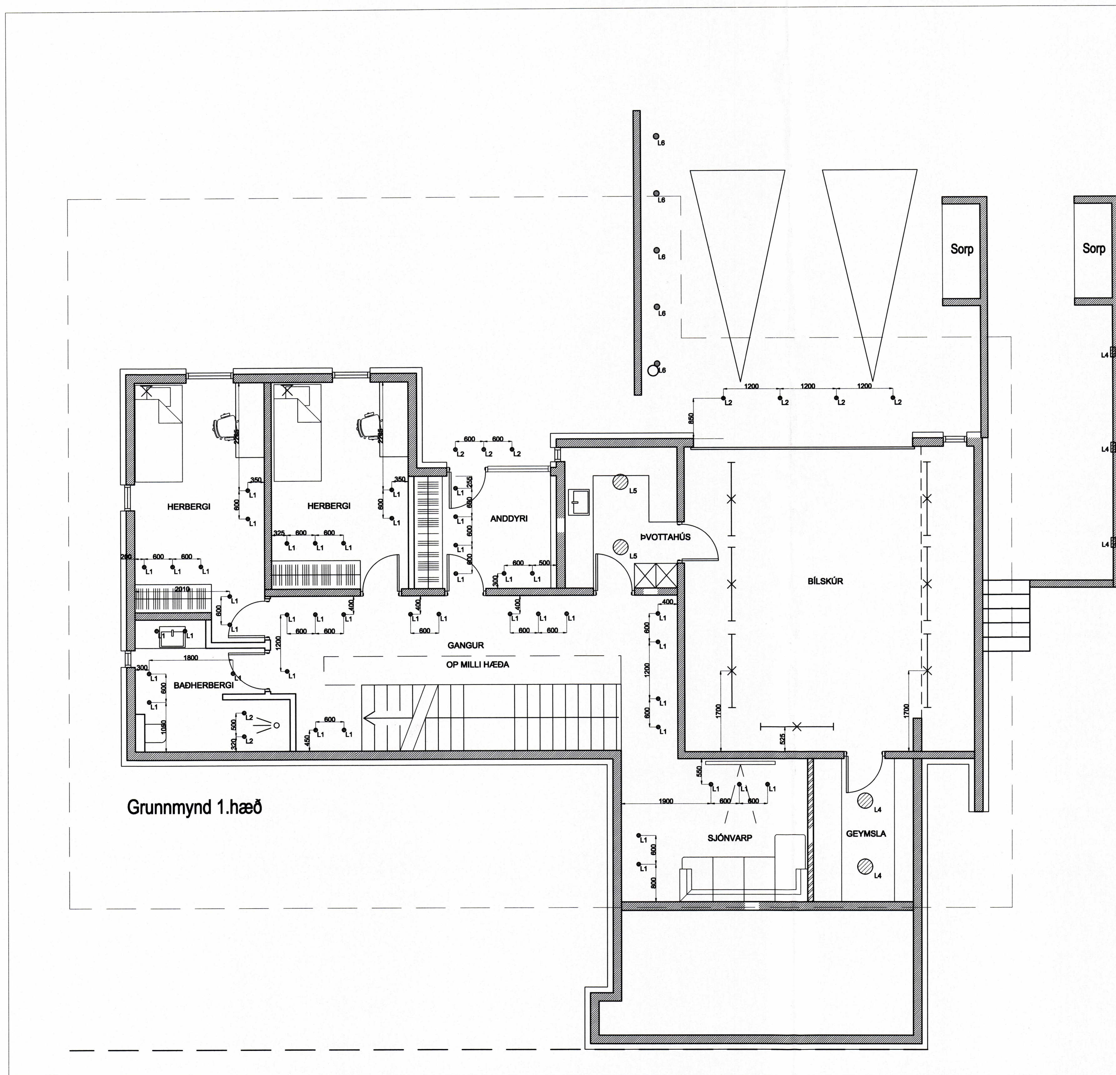
GRUNNMYND 1:50
