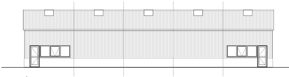
Útlit - norðurhlíð M 1:100
