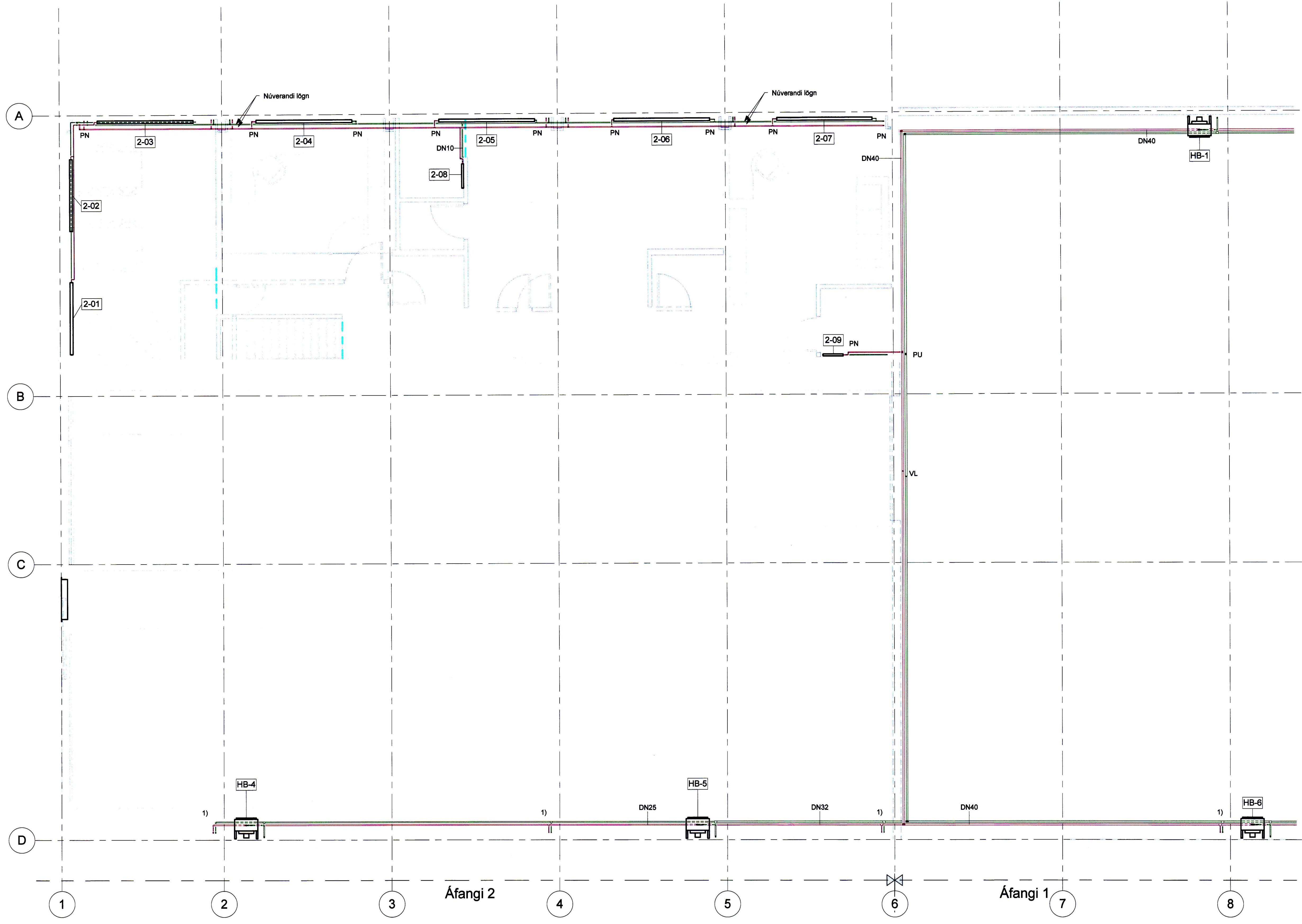
1 Grunnmynd 2. hæð 1 : 50
