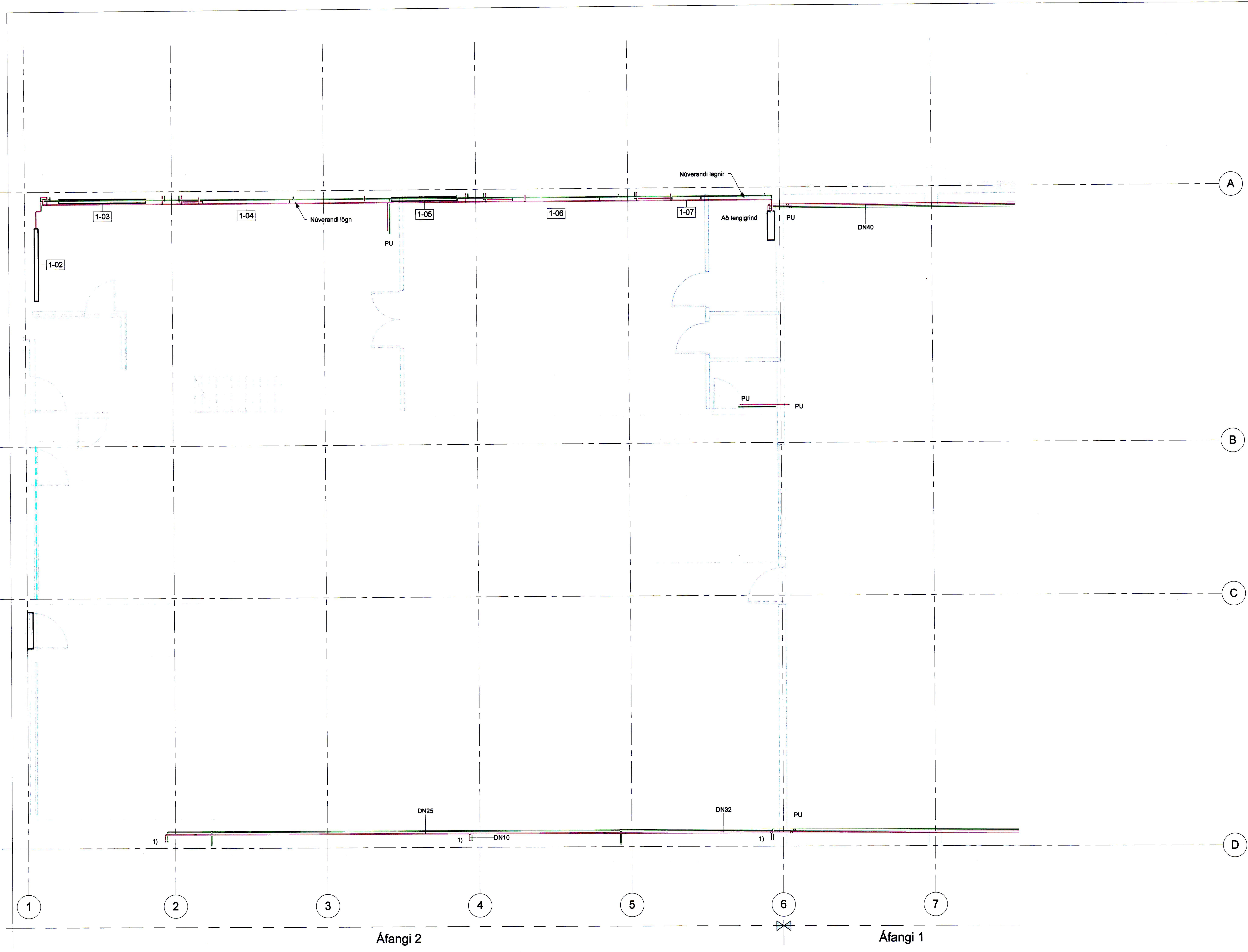
1 Grunnmynd 1.hæð 1 : 50
