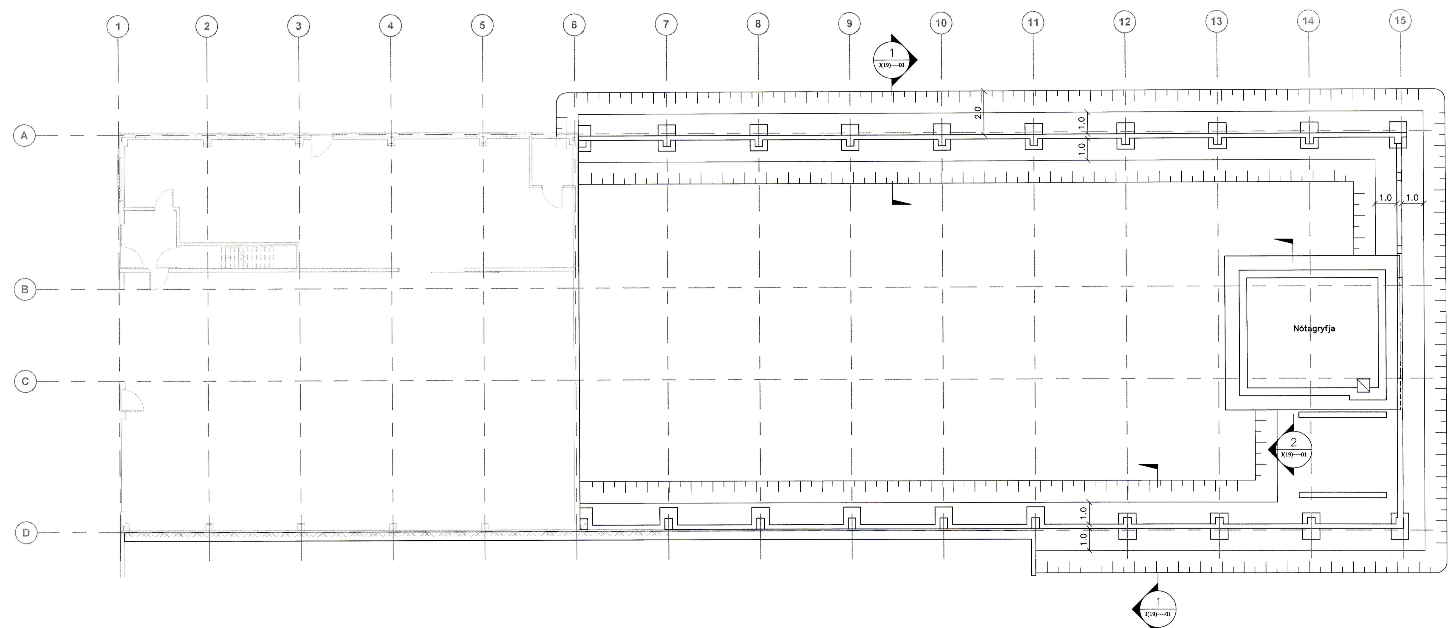
Grunnmynd graftarplans Mkv: 1:100
