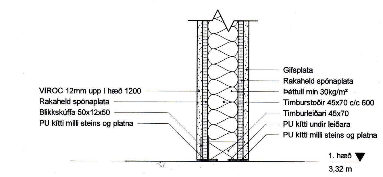
3 (41) - LÓ - Veggur að neðan 1:5
