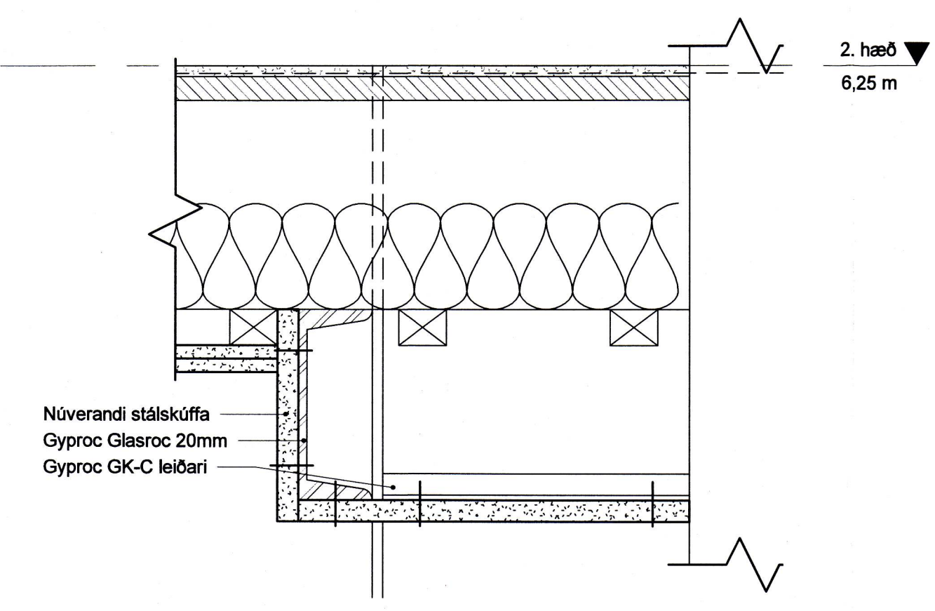
2 (45) LÓ - Frágangur við útvegg 1:5
