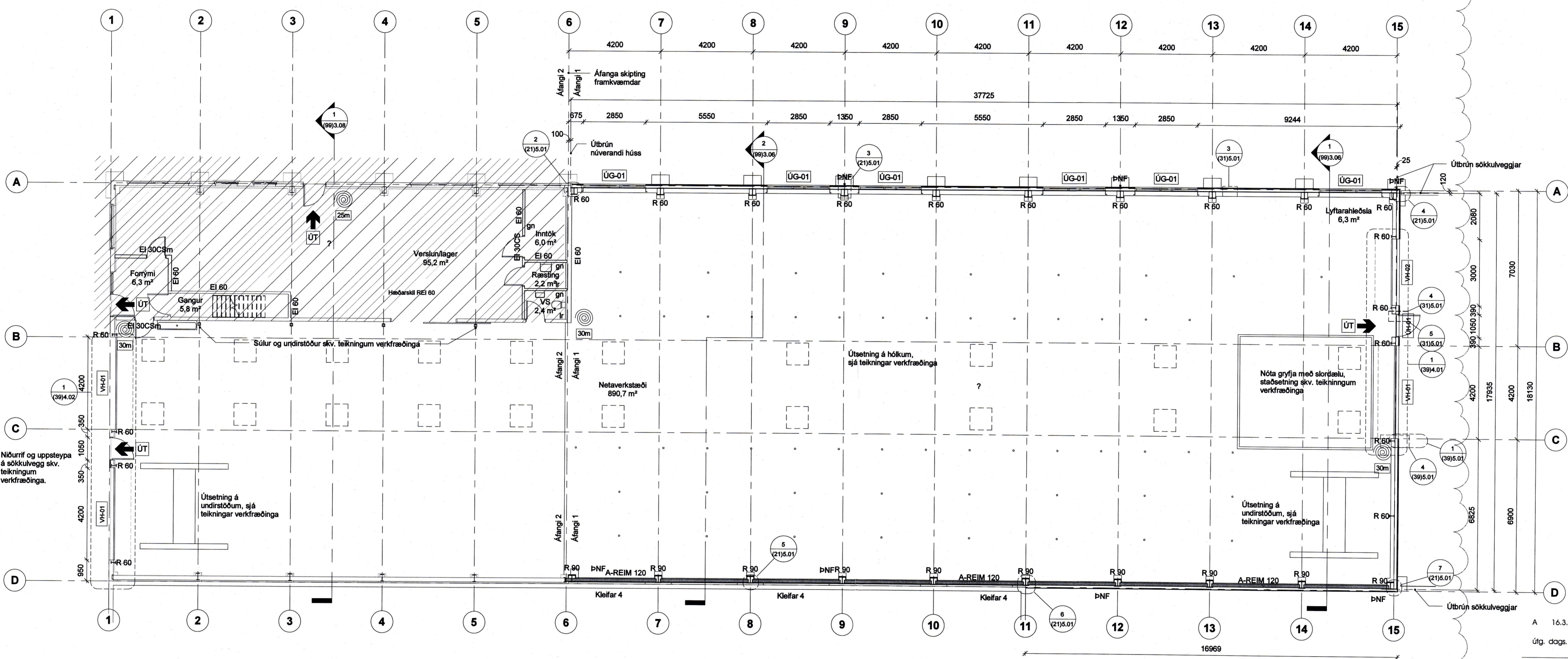
1 (99) Grunnmynd, 1. hæð 1 : 100
