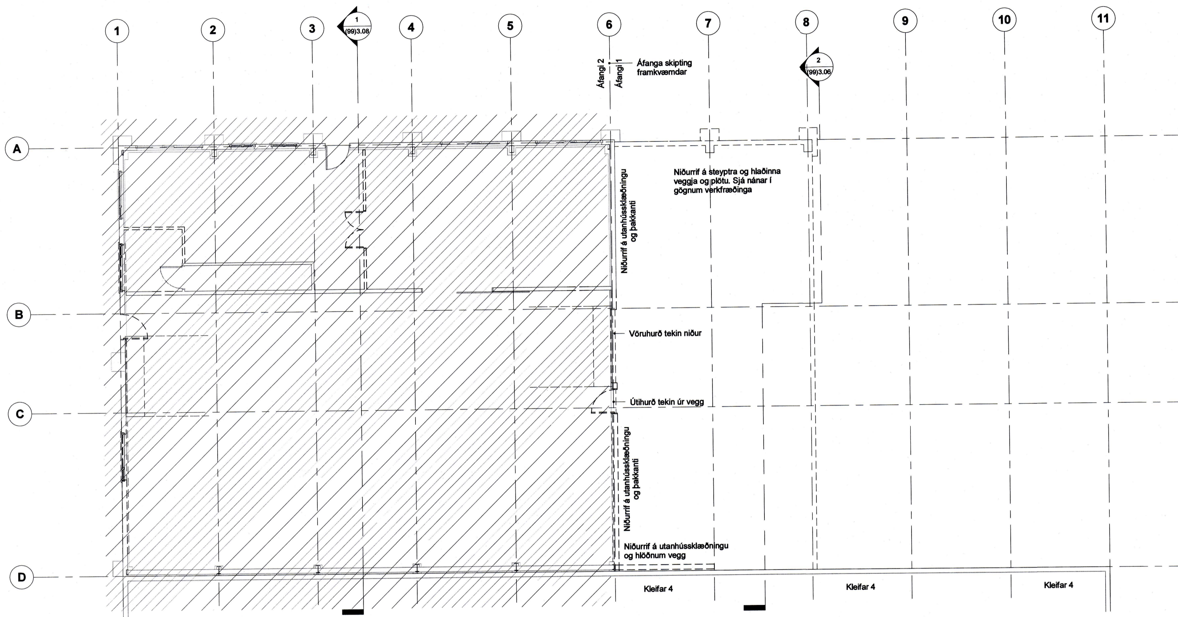
1 (98) Grunnmynd, 1. hæð - Niðurrif 1:100
