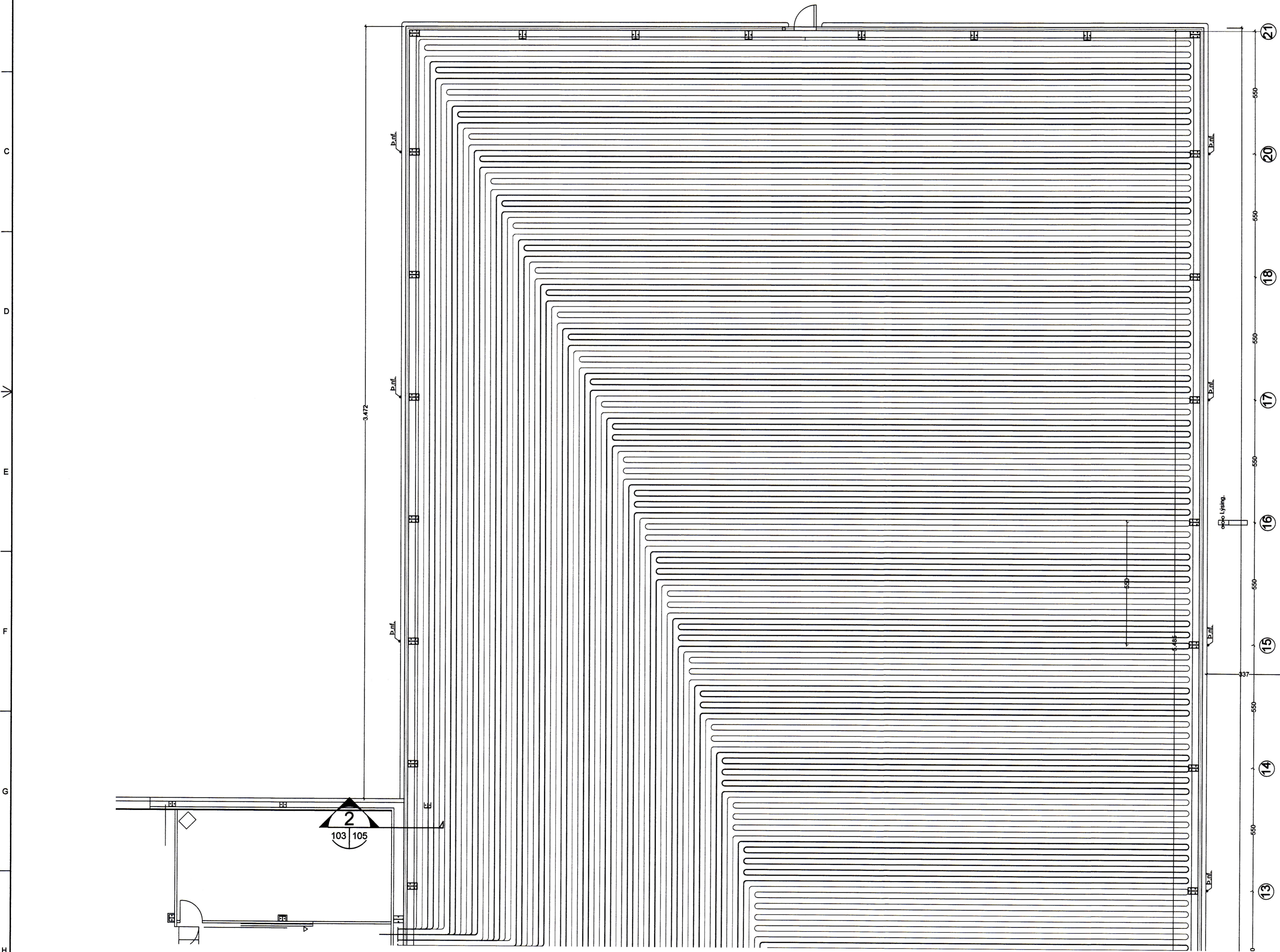
1 Grunnmynd 1 : 100
