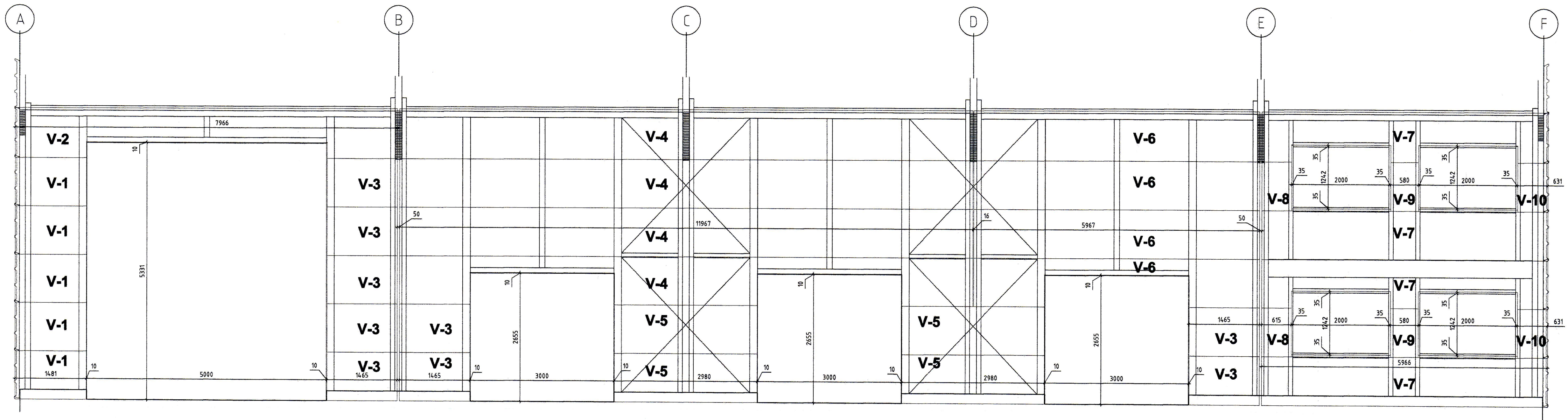
HLIDARMYND VESTUR Mkv 1:50
