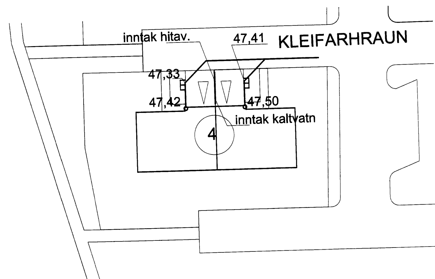
AFSTÖÐUMYND 1:500
