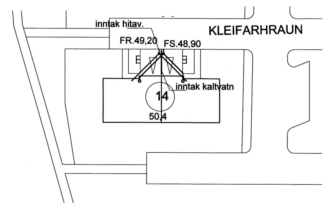
AFSTÖÐUMYND 1:500
