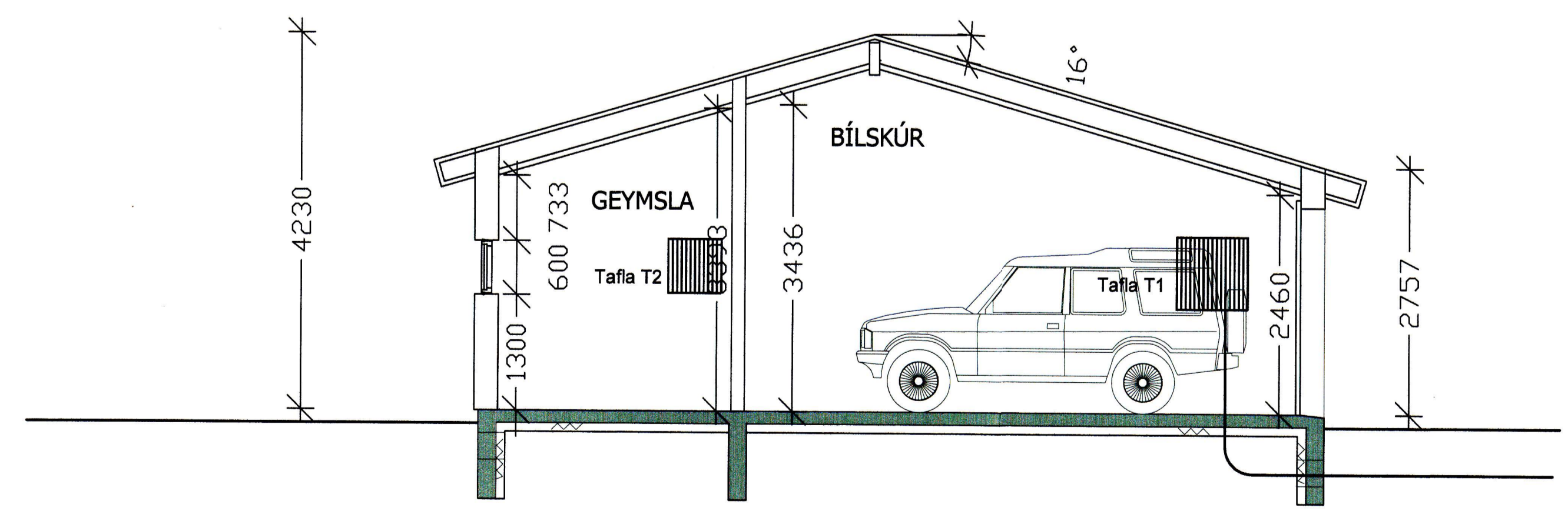
SNIÐ B-B
