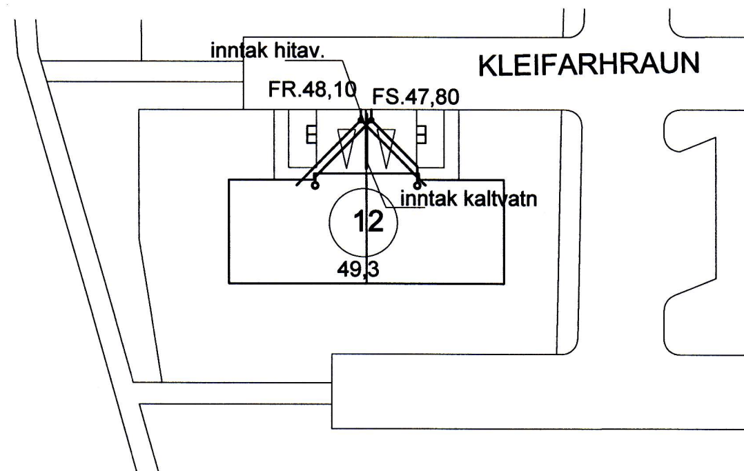
AFSTÖÐUMYND 1:500
