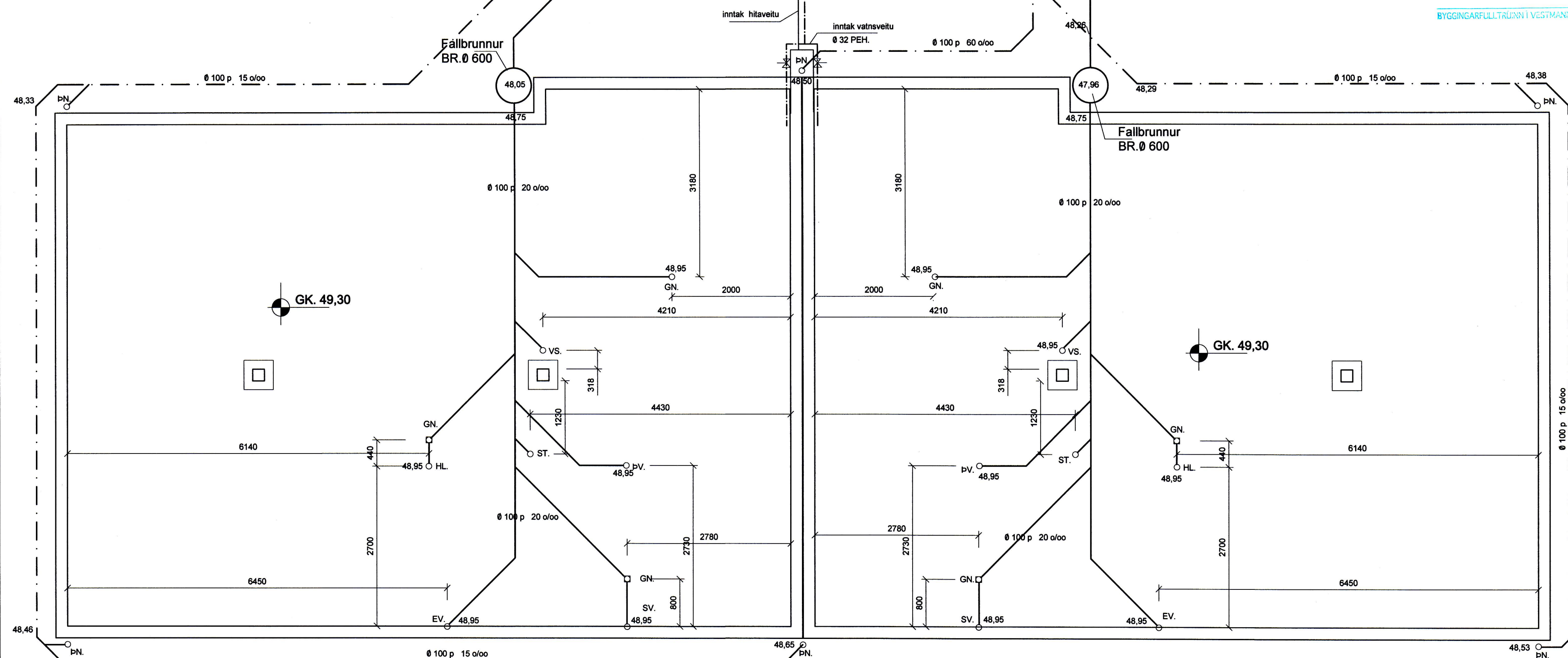
AFSTÖÐUMYND 1:500
