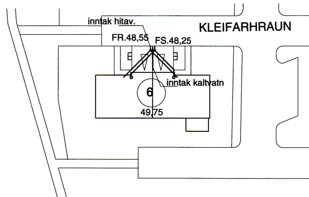
AFSTÖÐUMYND 1:500
