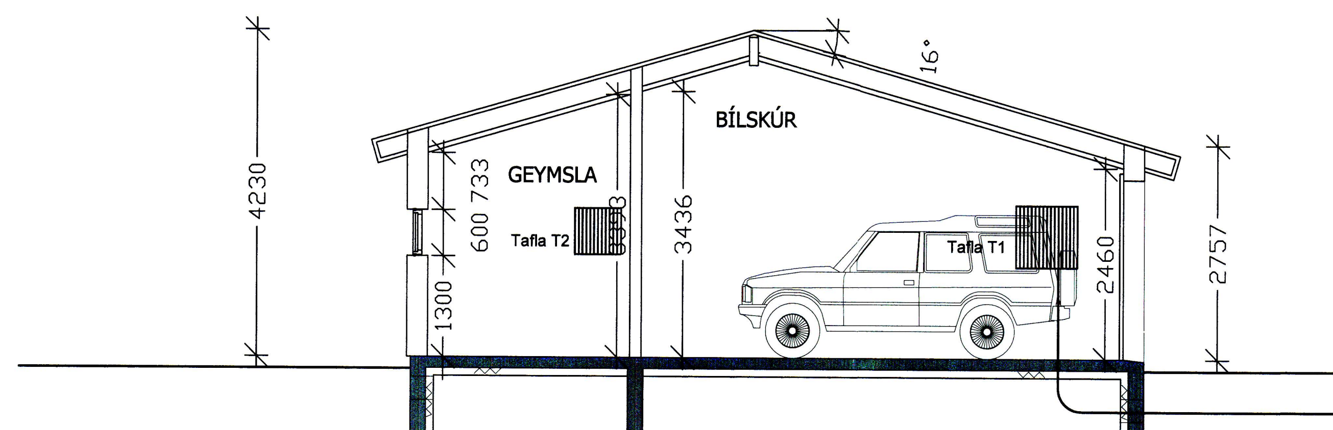
SNIÐ B-B
