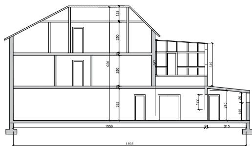
Snið B-B
