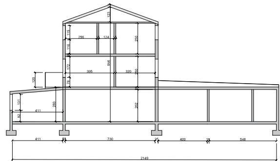
Snið A-A
