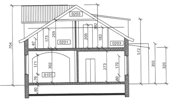
SNID A-A
