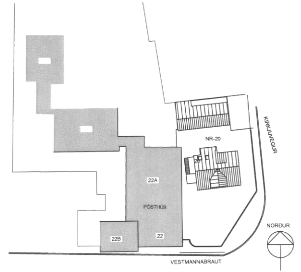
AFSTÖÐUMYND M=500
