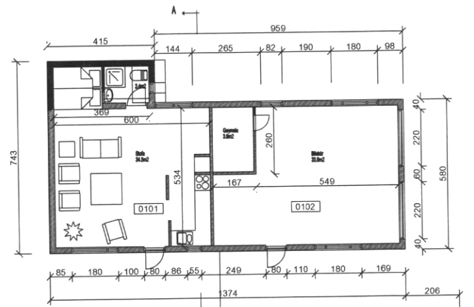
GRUNNMYND BILSKUR
