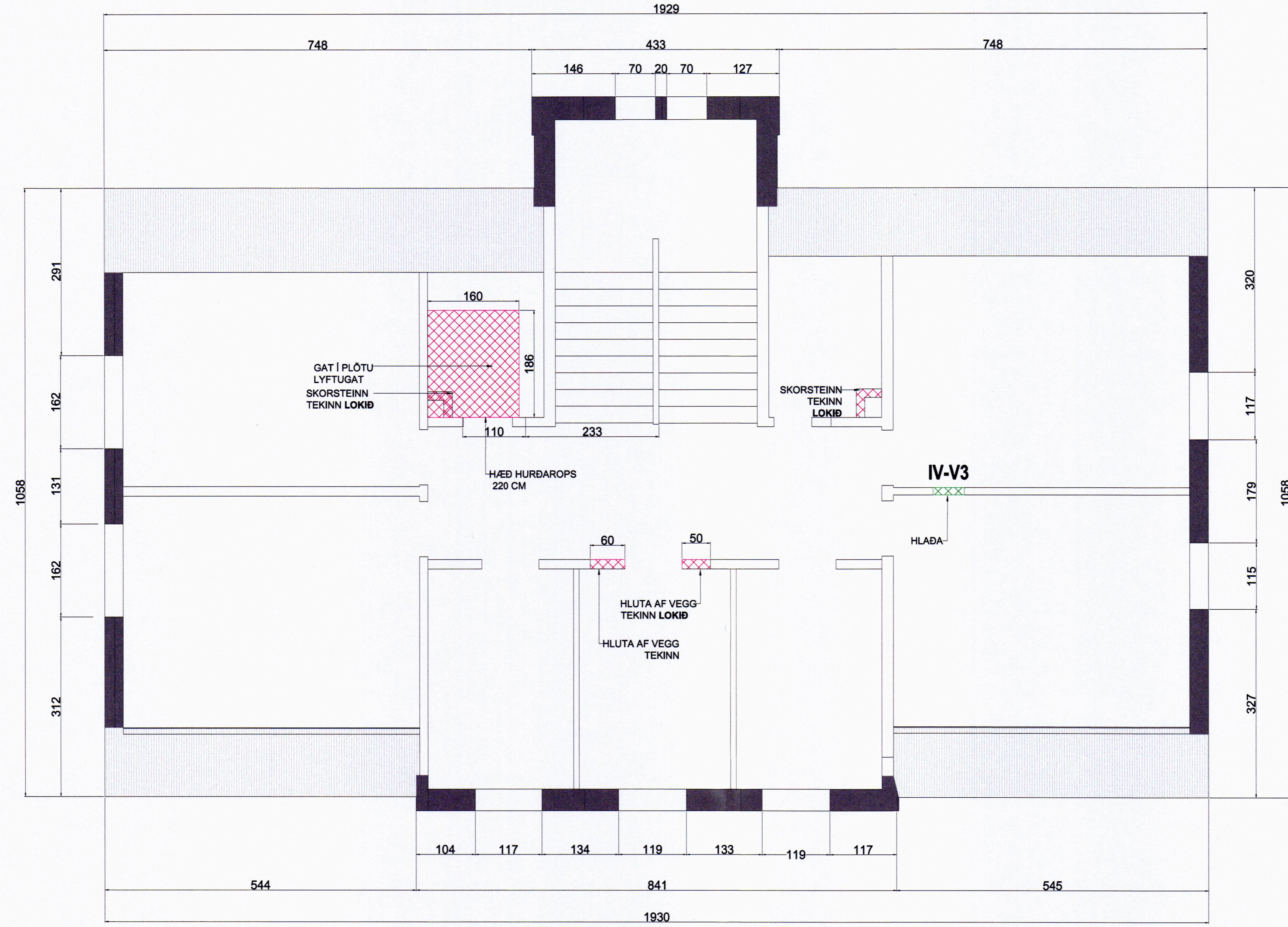
GRUNNMYND 2 HÆÐ
