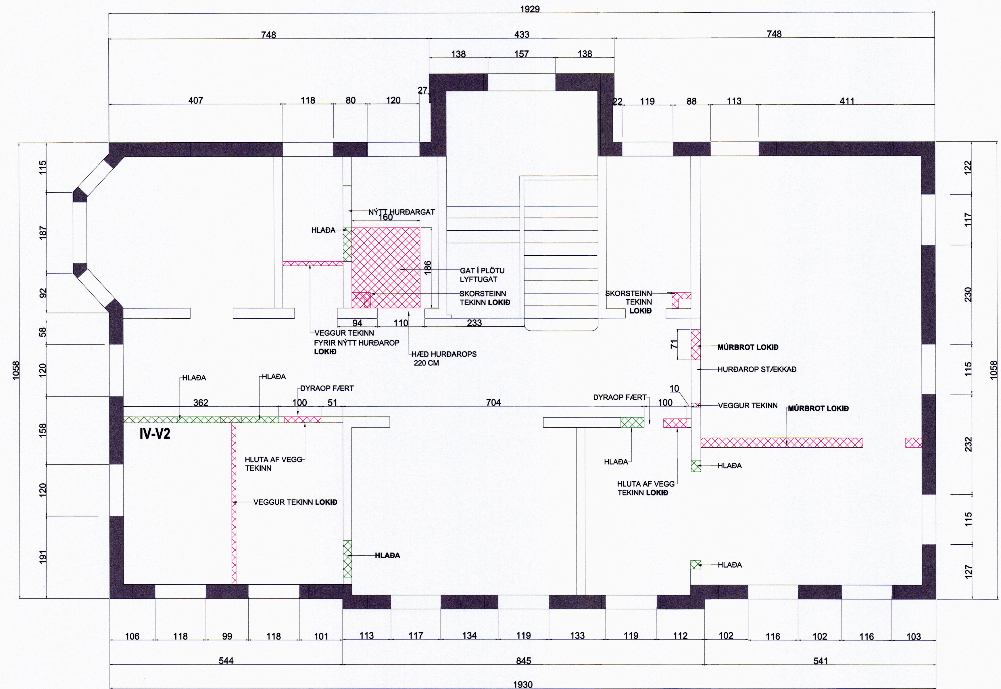
GRUNNMYND 1 HÆÐ
