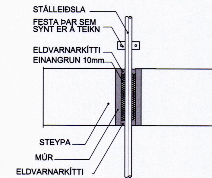
FRÁGANGUR Á STÁLLEIÐSLU GEGNUM STEYPT GÓLF
