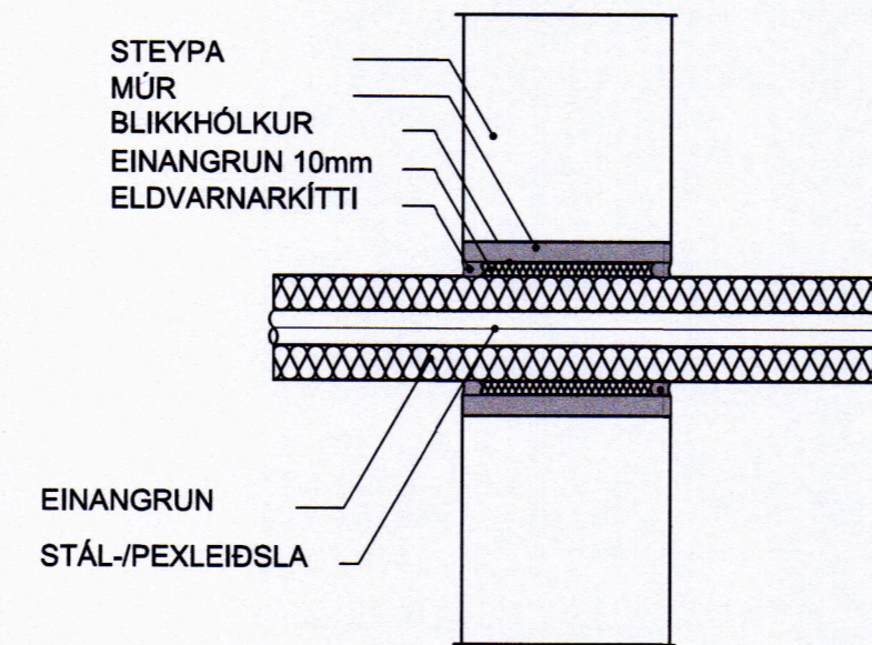
FRÁGANGUR Á STÁL-/PEKLEIÐSLU GEGNUM STEYPTAN VEGG
