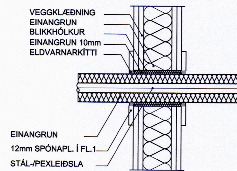
FRÁGANGUR Á STÁL-/PEKLEIÐSLU GEGNUM LÉTTAN VEGG
