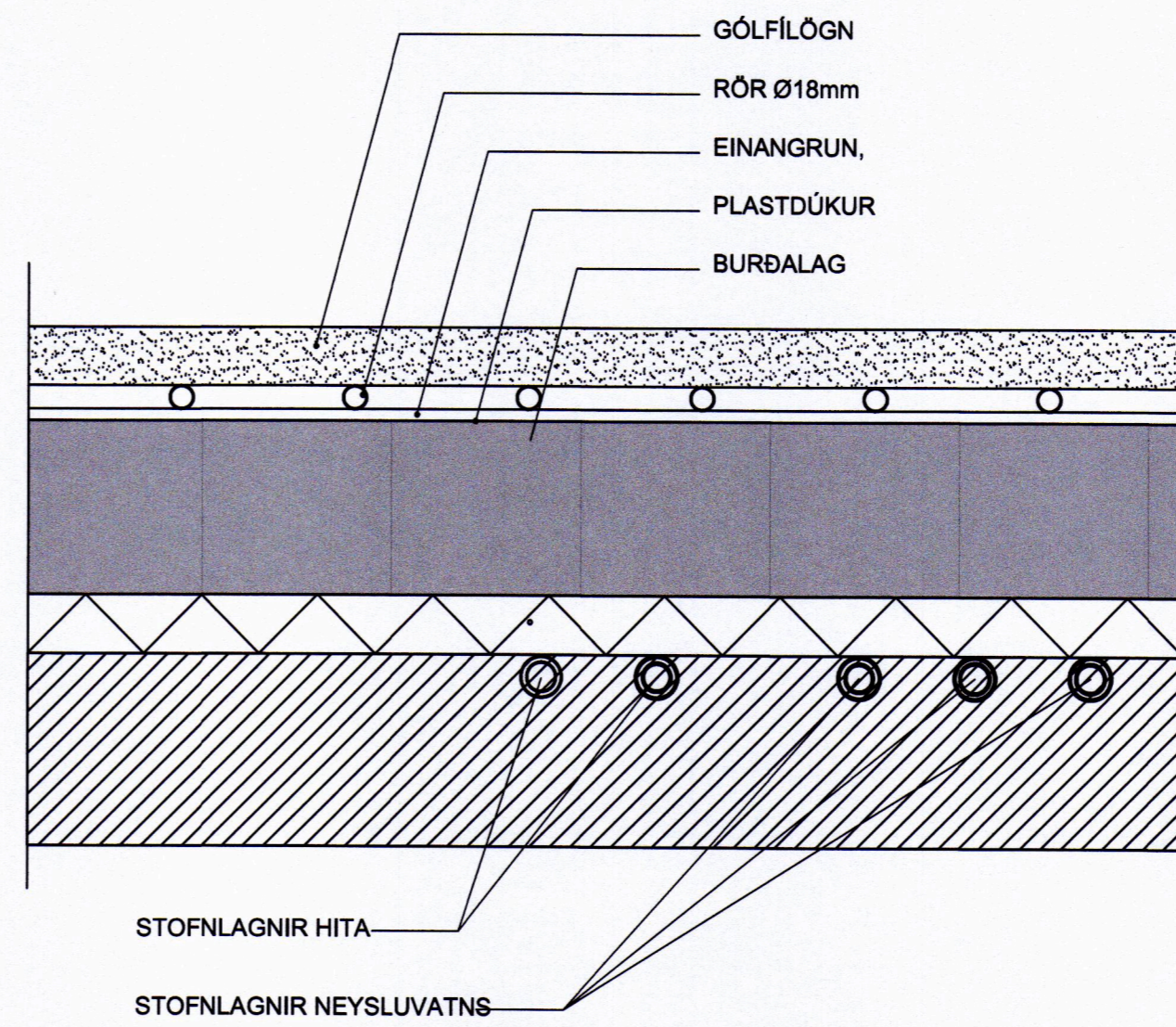
FRÁGANGUR LAGNA Í GÓLFI
