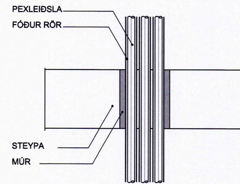
FRÁGANGUR Á PEKLEIÐSLU GEGNUM STEYPT GÓLF
