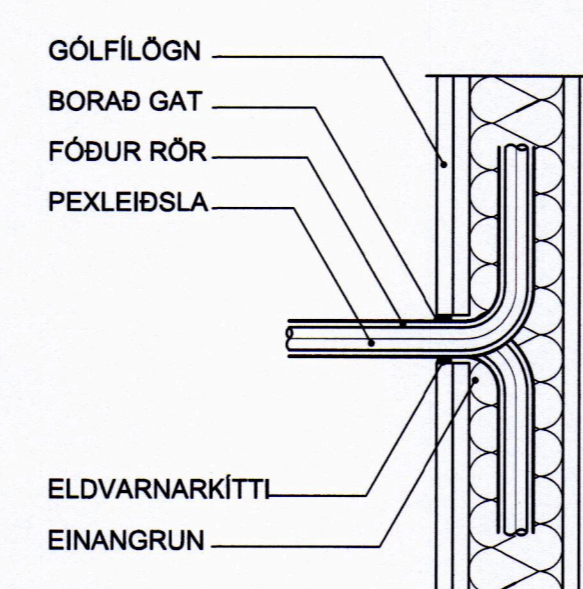
BRUNAPÉTTING Á PEKLEIÐSLU Í FÓÐURRÖRI Í GEGNUM KLÆÐNINGU
