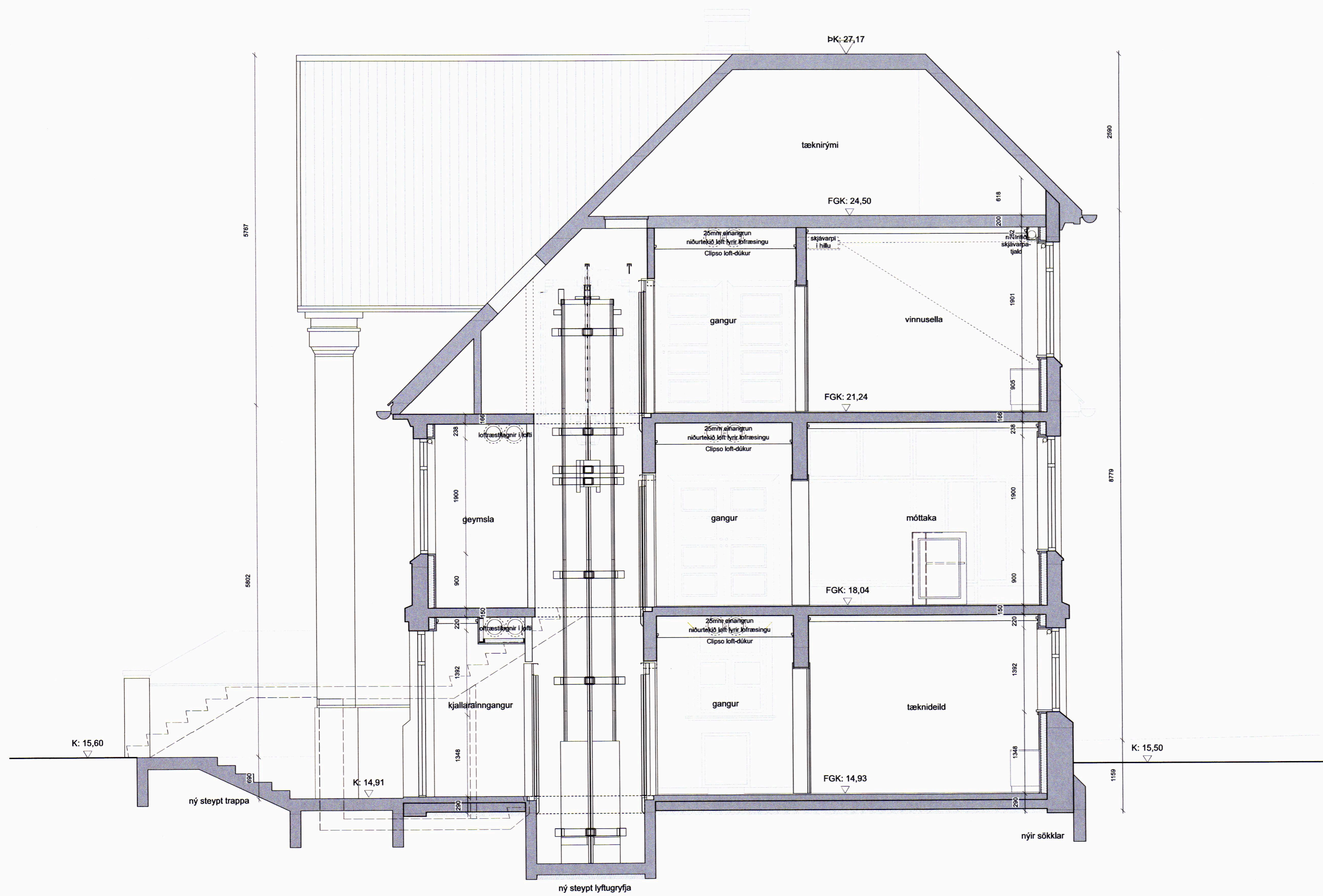
Sneiðing D-D
