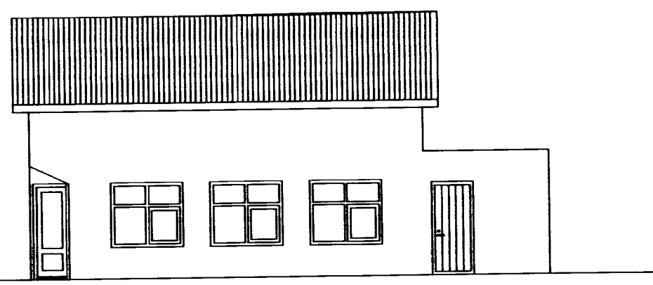
útlit suður mkv 1:100
