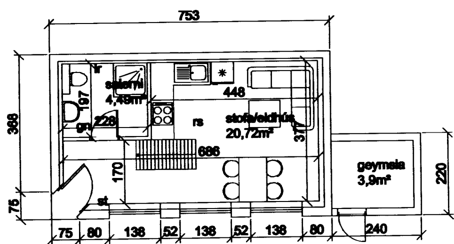
grunnmynd neðri hæð mkv 1:100
