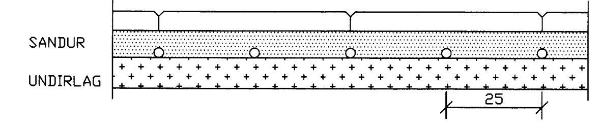
FRÁGANGUR RÖRA UNDIR HELLULÖGN M=1:10
