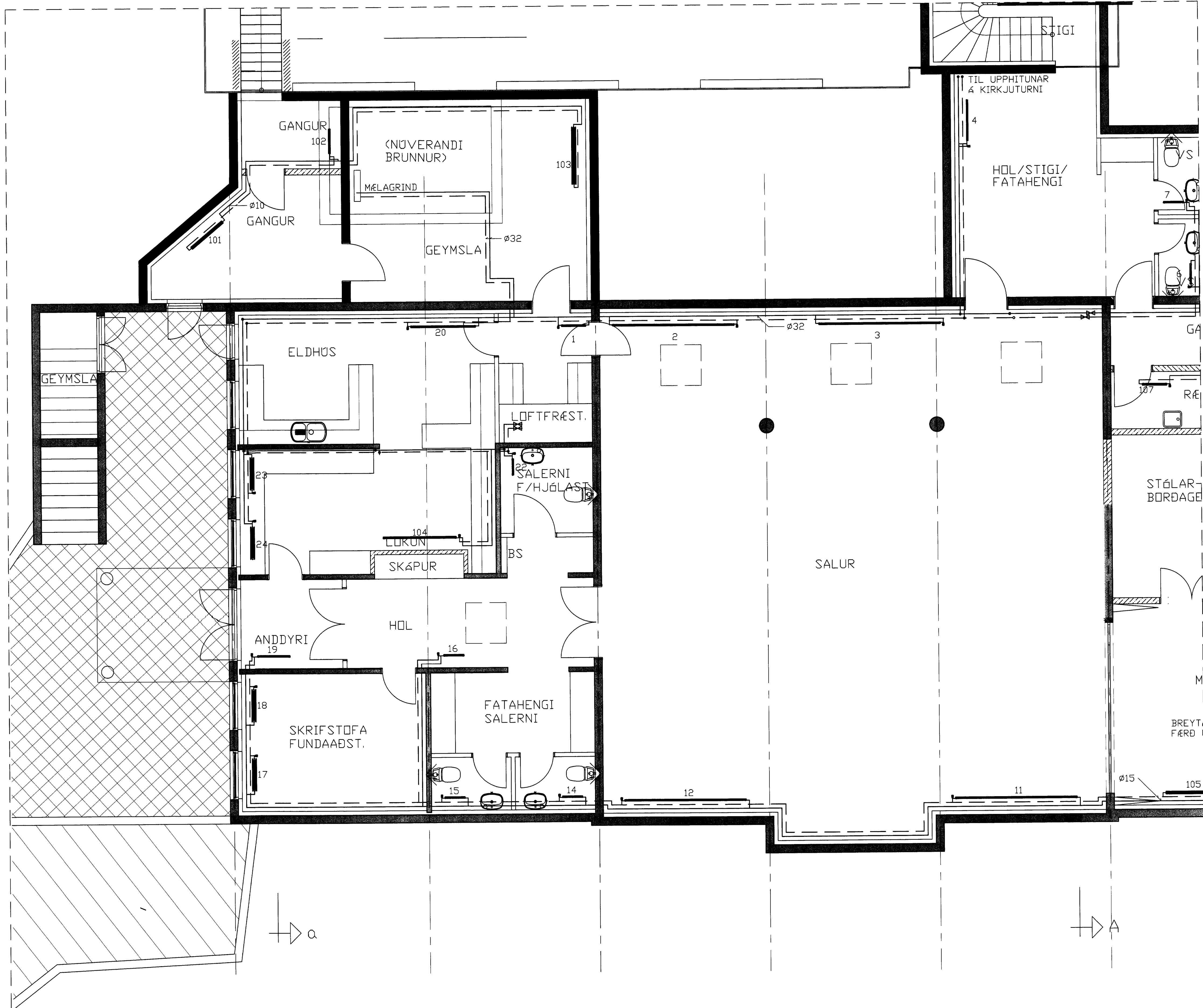
GRUNNMYND AUSTURENDI M=1:50
