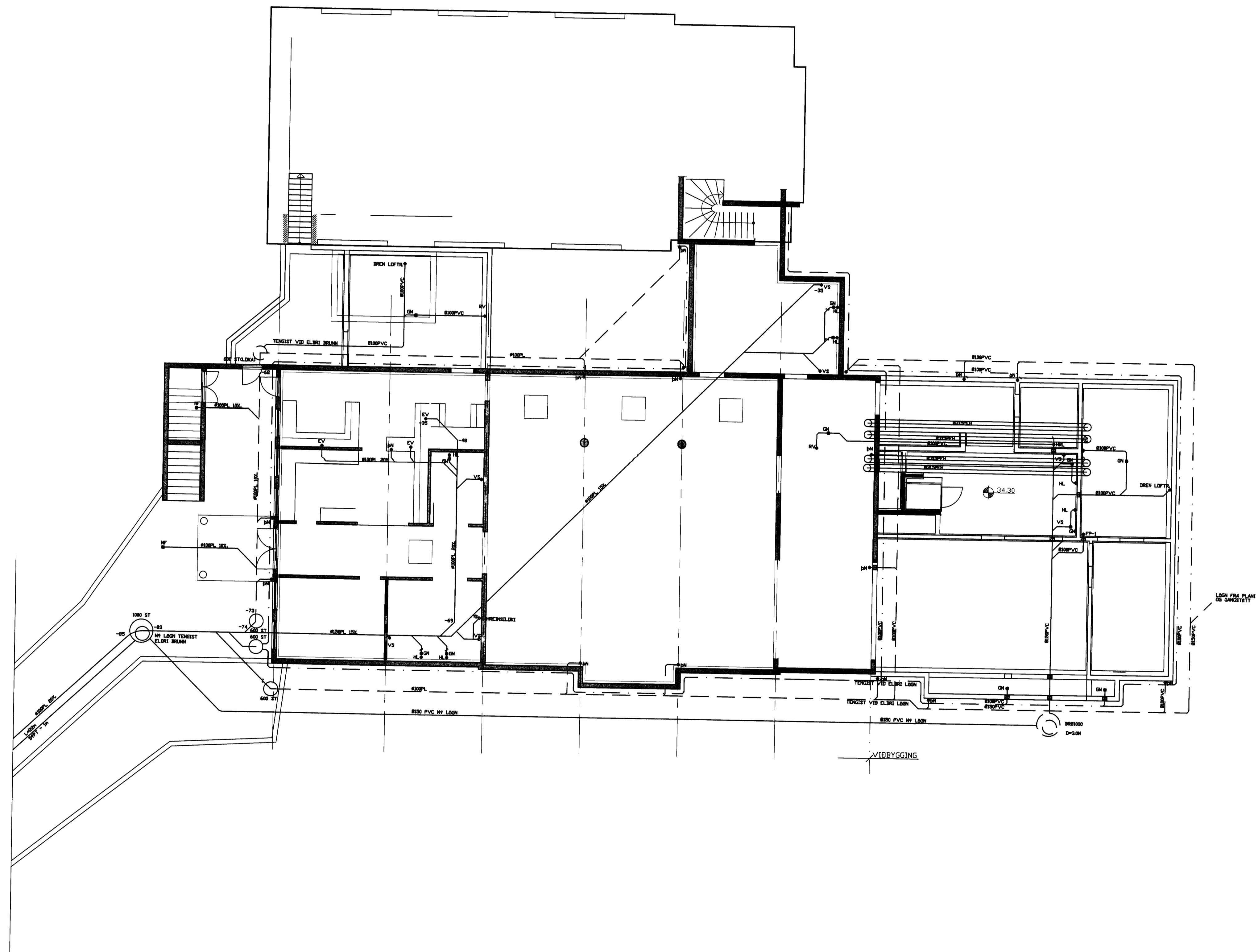
GRUNNMYND UNDIRSTÖÐUR M=1:50
