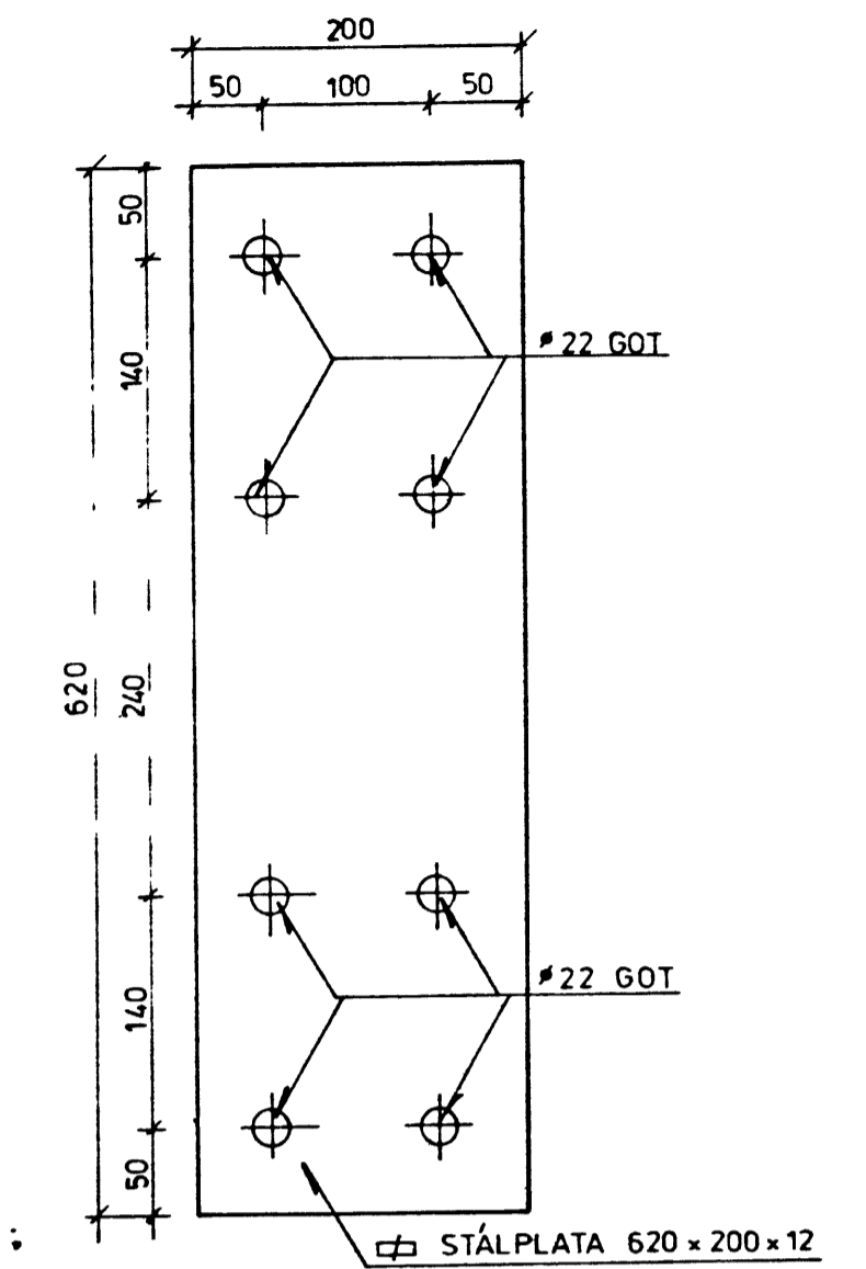
FESTING NR. 5 2 stk. SJÁ DEILI N, TEIKN. NR. 542-520
