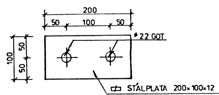
FESTING NR. 9 4 stk. SJÁ DEILI A, TEIKN. NR. 542-527
