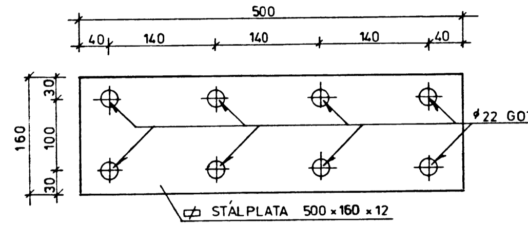
FESTING NR. 3 8 stk. SJÁ DEILI E, TEIKN NR. 542-528
