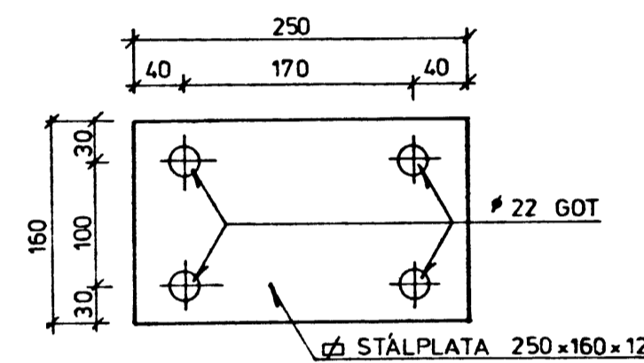
FESTING NR. 7 36 stk. SJÁ DEILI B, TEIKN. NR. 542-527 DEILI D, TEIKN. NR. 542-528 DEILI G, TEIKN. NR. 542-529
