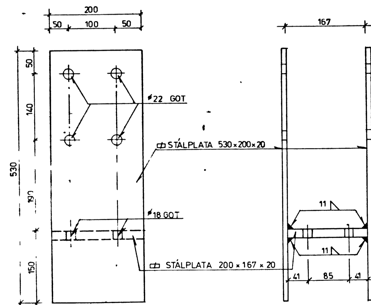
FESTING NR. 8 2 stk. SJÁ DEILI O, TEIKN. NR. 542-520
