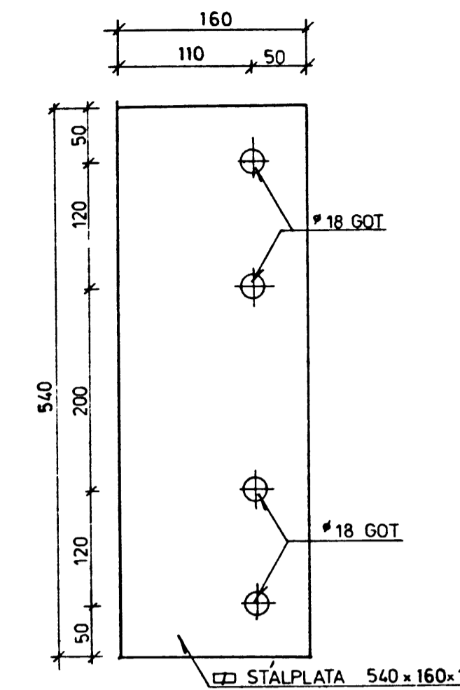
FESTING NR. 4 6 stk. SJÁ DEILI P, TEIKN. NR. 542-521
