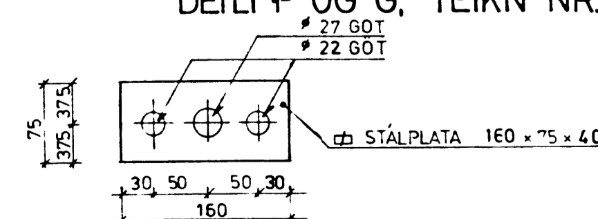
FESTING NR. 10 44 stk. SJÁ DEILI A, B OG C, TEIKN. NR. 542-527 DEILI D OG E, TEIKN. NR. 542-528 DEILI F OG G, TEIKN. NR. 542-528
