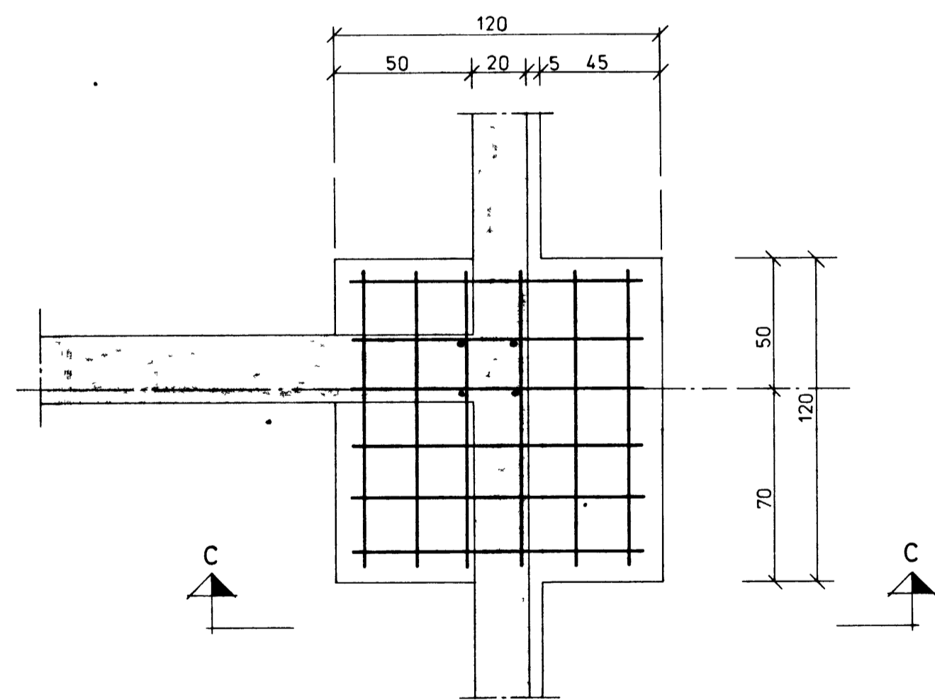
UNDIRSTAÐA U-6, GRUNNMYND, M 120
