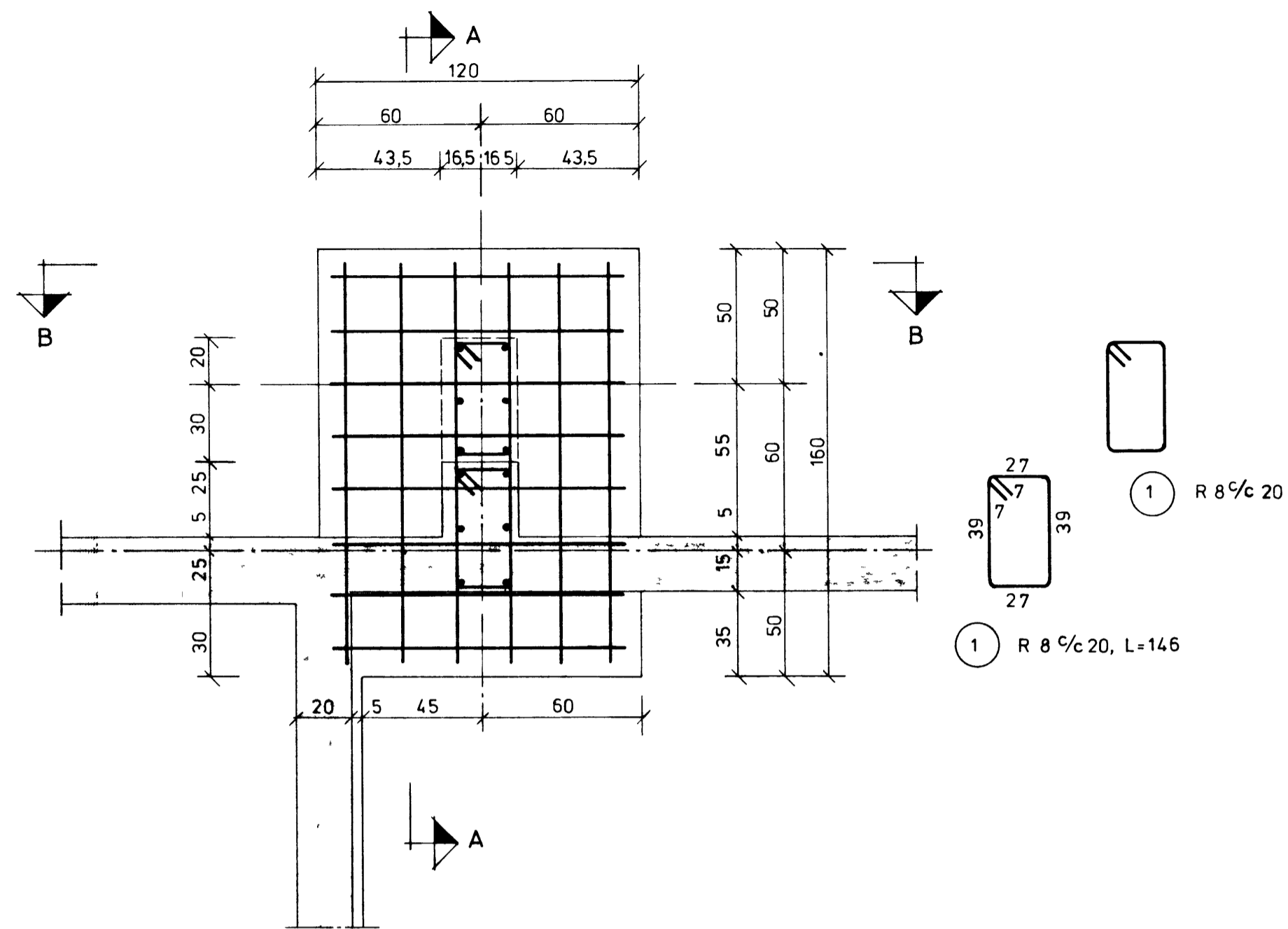
UNDIRSTAÐA U-5, M 120
