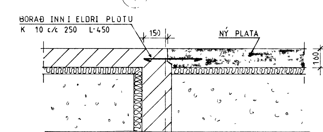
SNIÐ B 120
