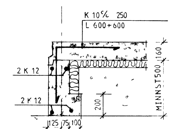
SNIÐ C 120
