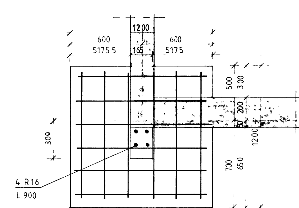
UNDIRSTÖÐUR U1 120
