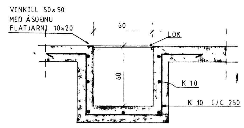
SNIÐ A-A 120
