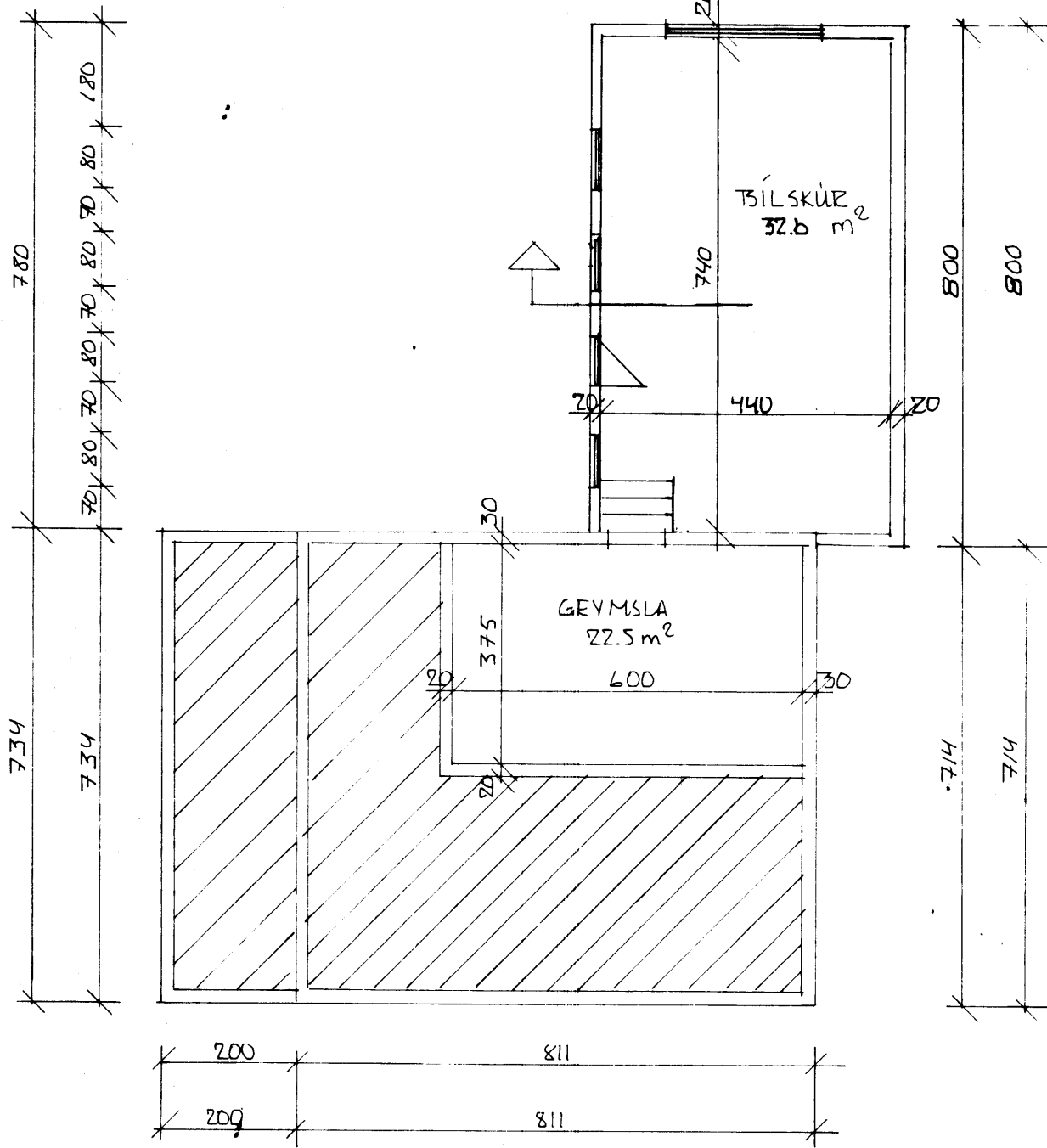
GRUNNMYND KJALLARI M=1:100
