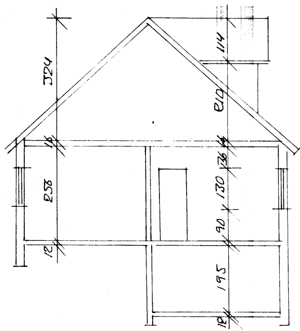
SNÍÐ A-A M=1:100
