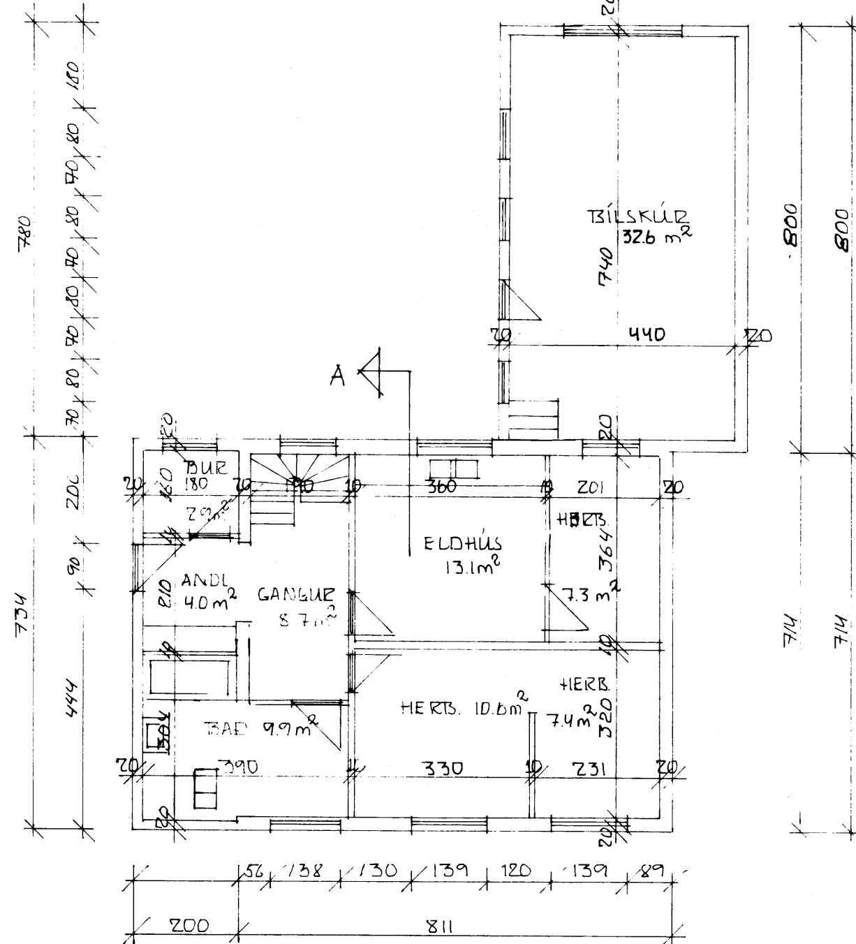
GRUNNMYND 1. HÆÐ M=1:100
