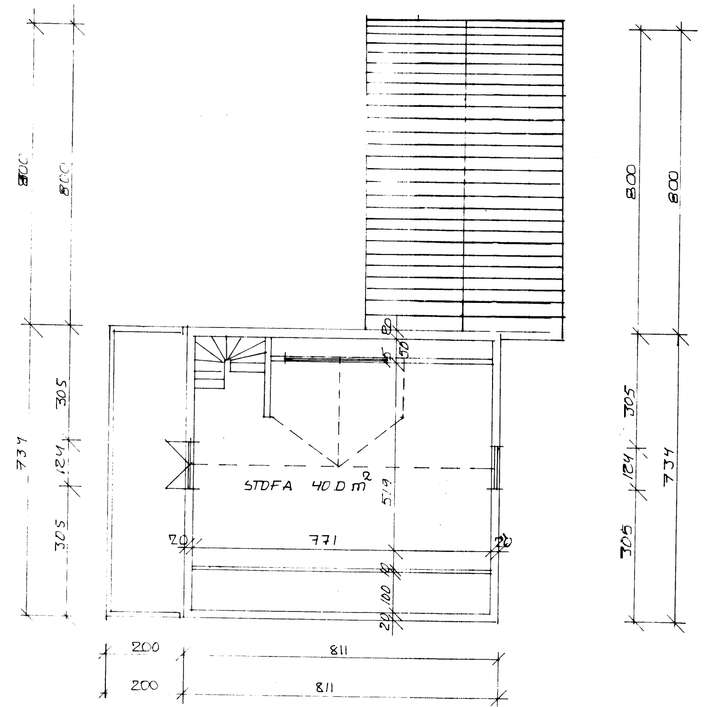
GRUNNMYND ÞLS M=1:100
