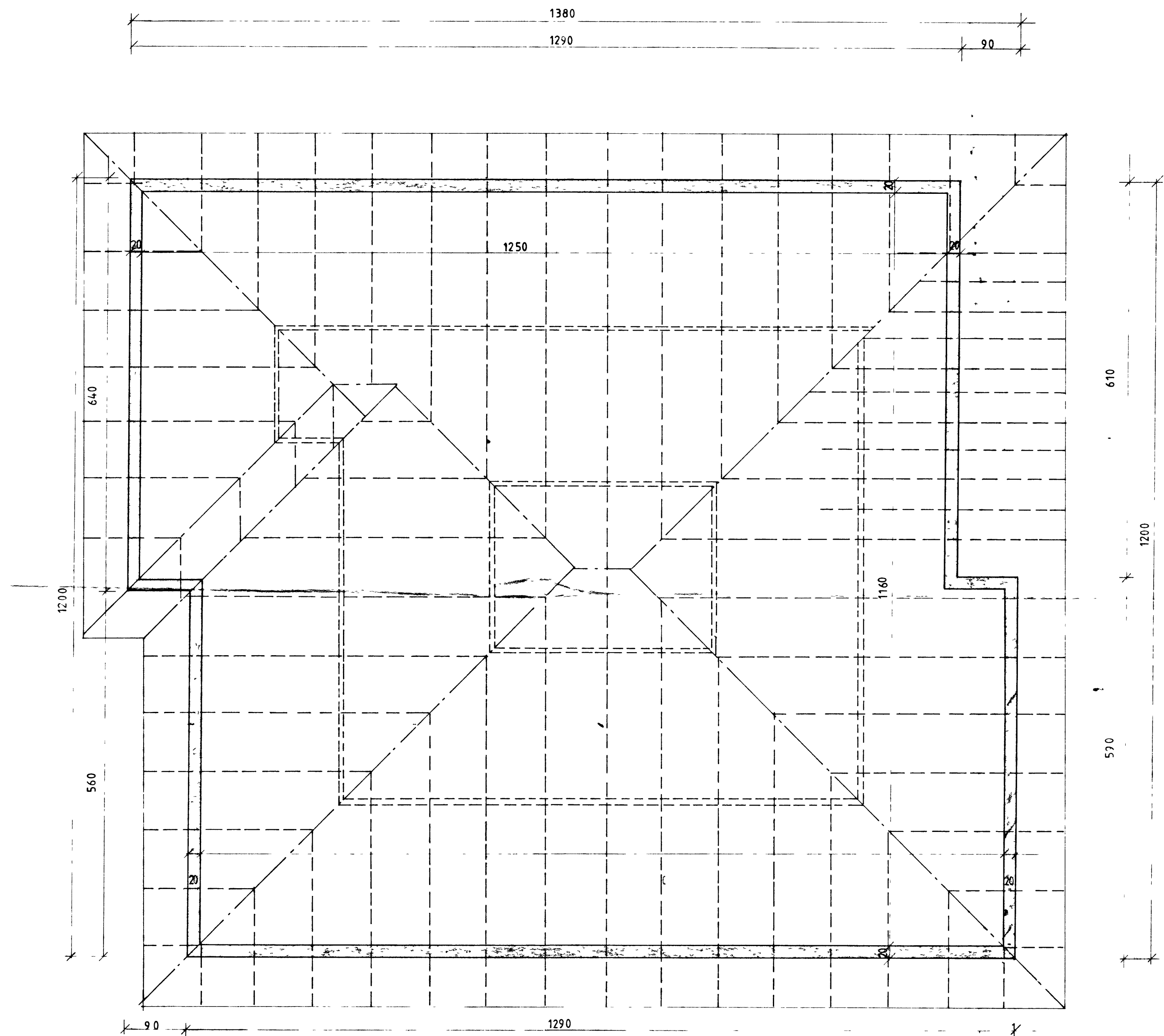
Grunnmynd Pak 1:50
