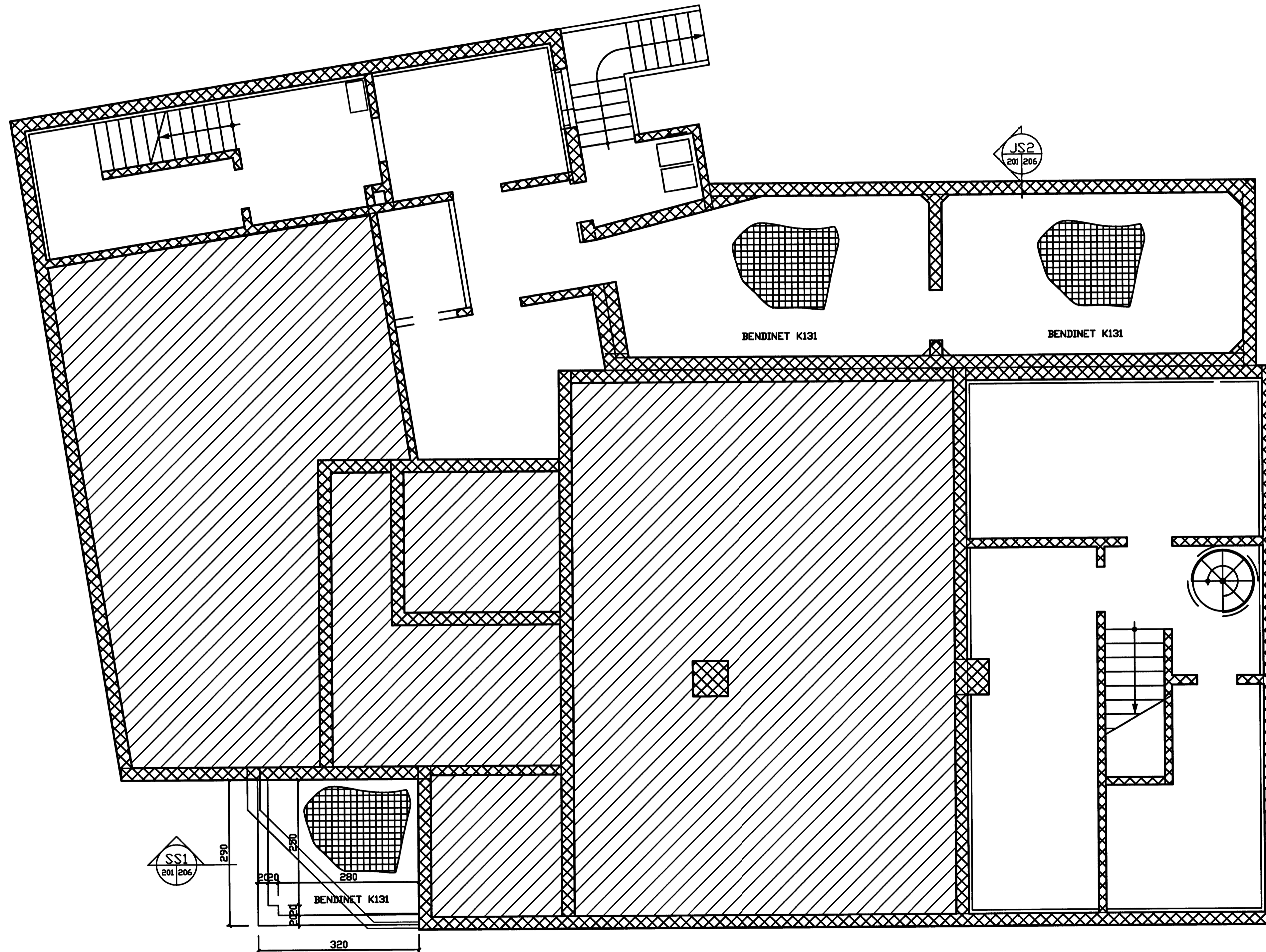
GRUNNMYND KJALLARI M=1:50
