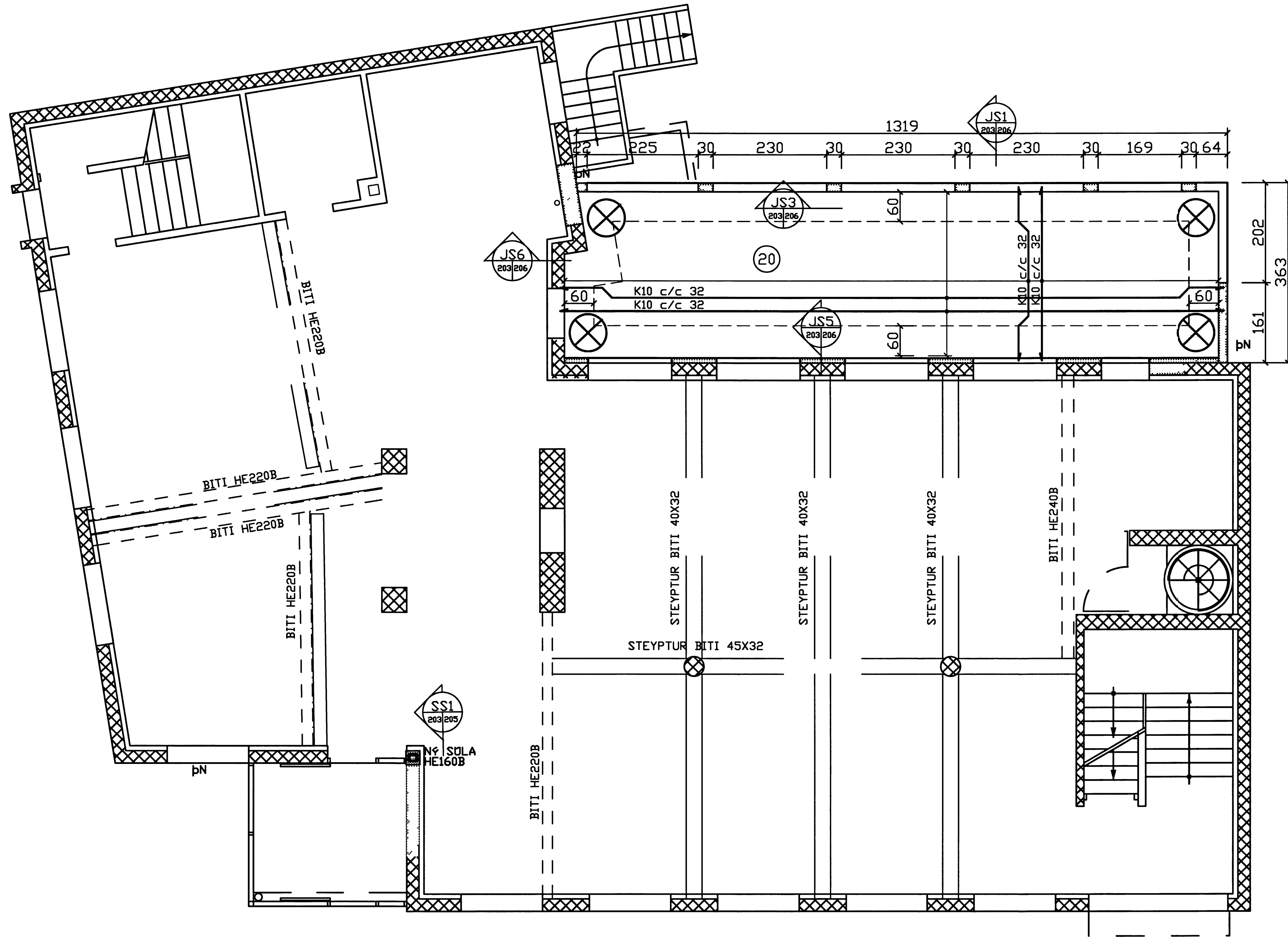
GRUNNMYND 1. HÆÐ M=1/50
