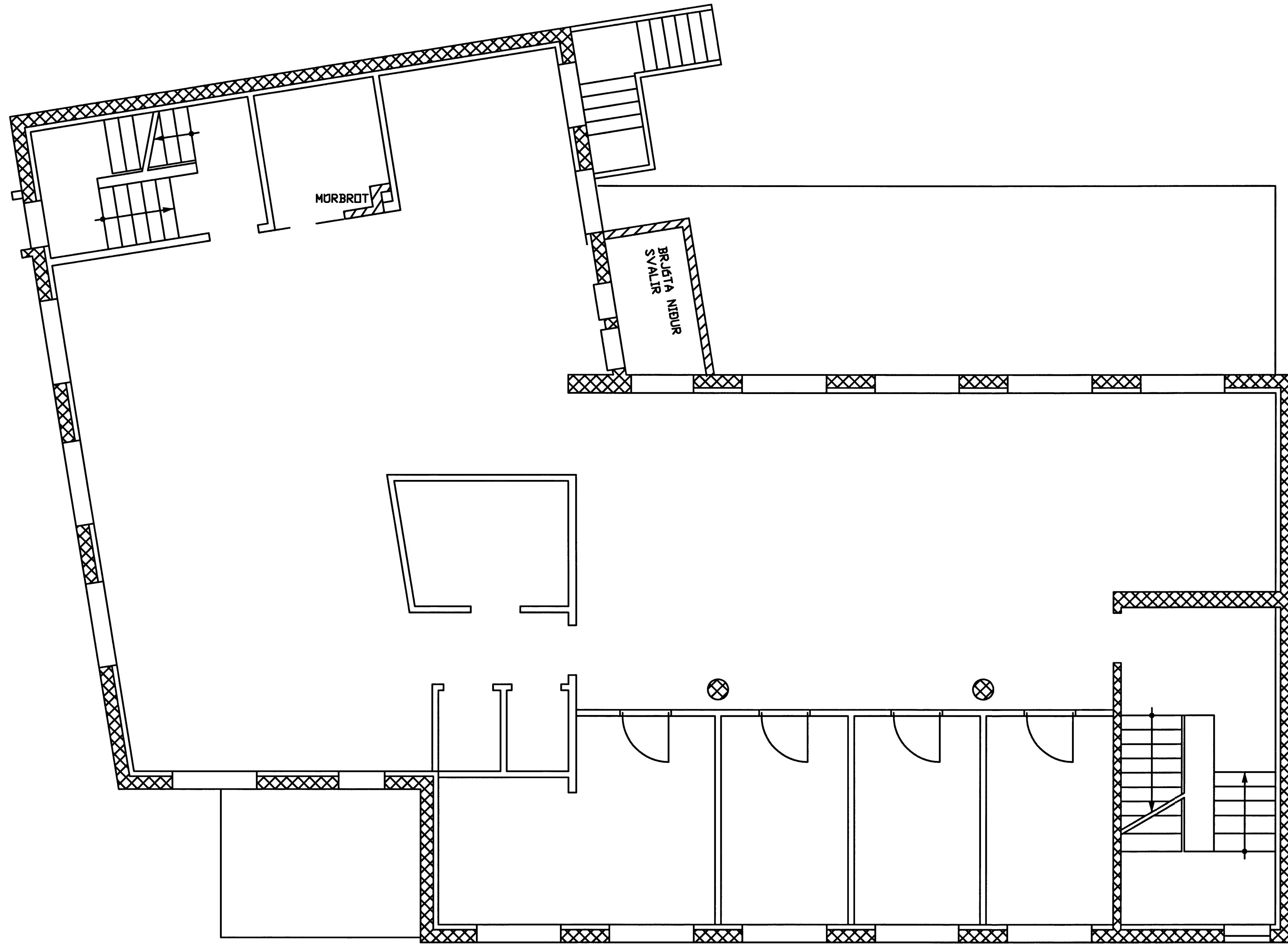
GRUNNMYND 2. HÆÐ M=1:50
