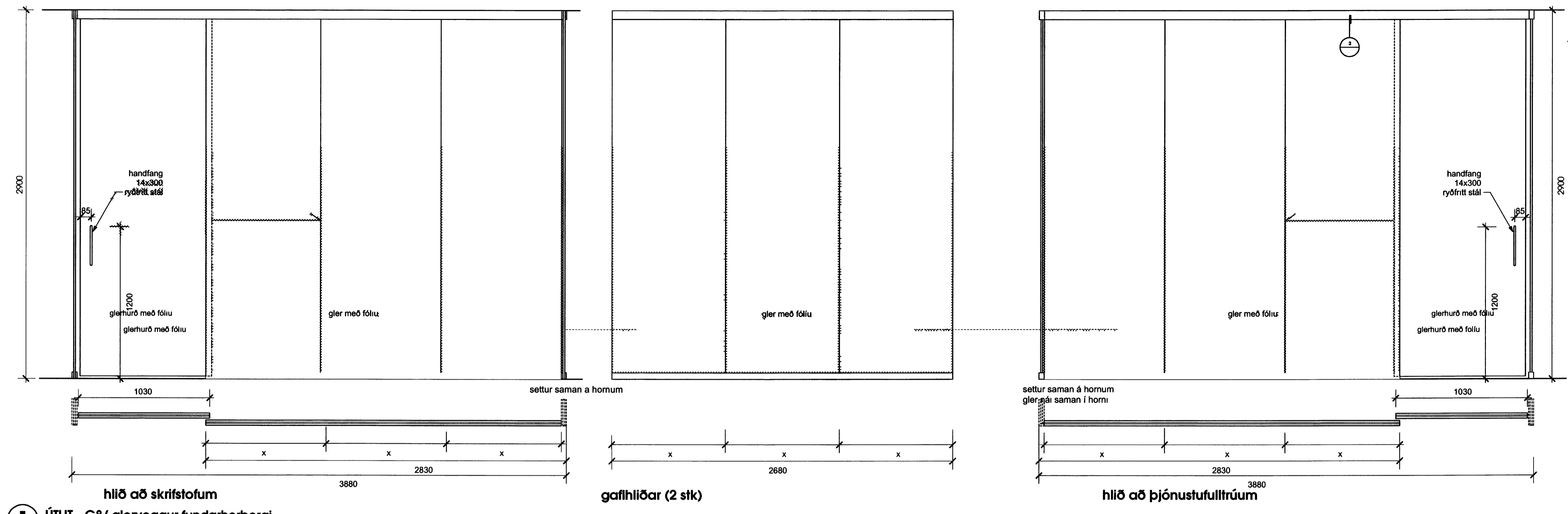
1 ÚTLIT - G8/ glerveggur fundarherbergi mív 1.20
