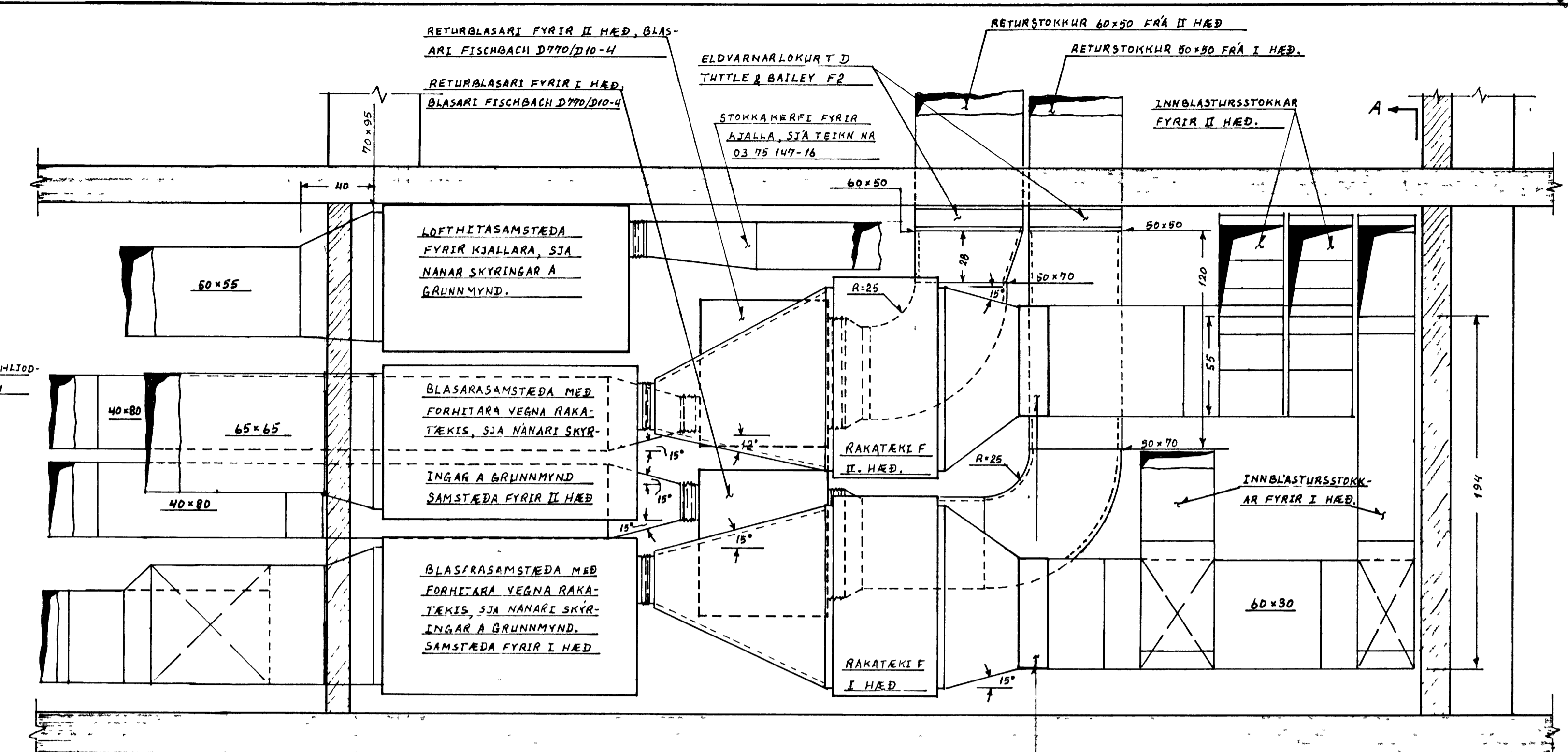
SNEIÐING B-B, 1:20.
