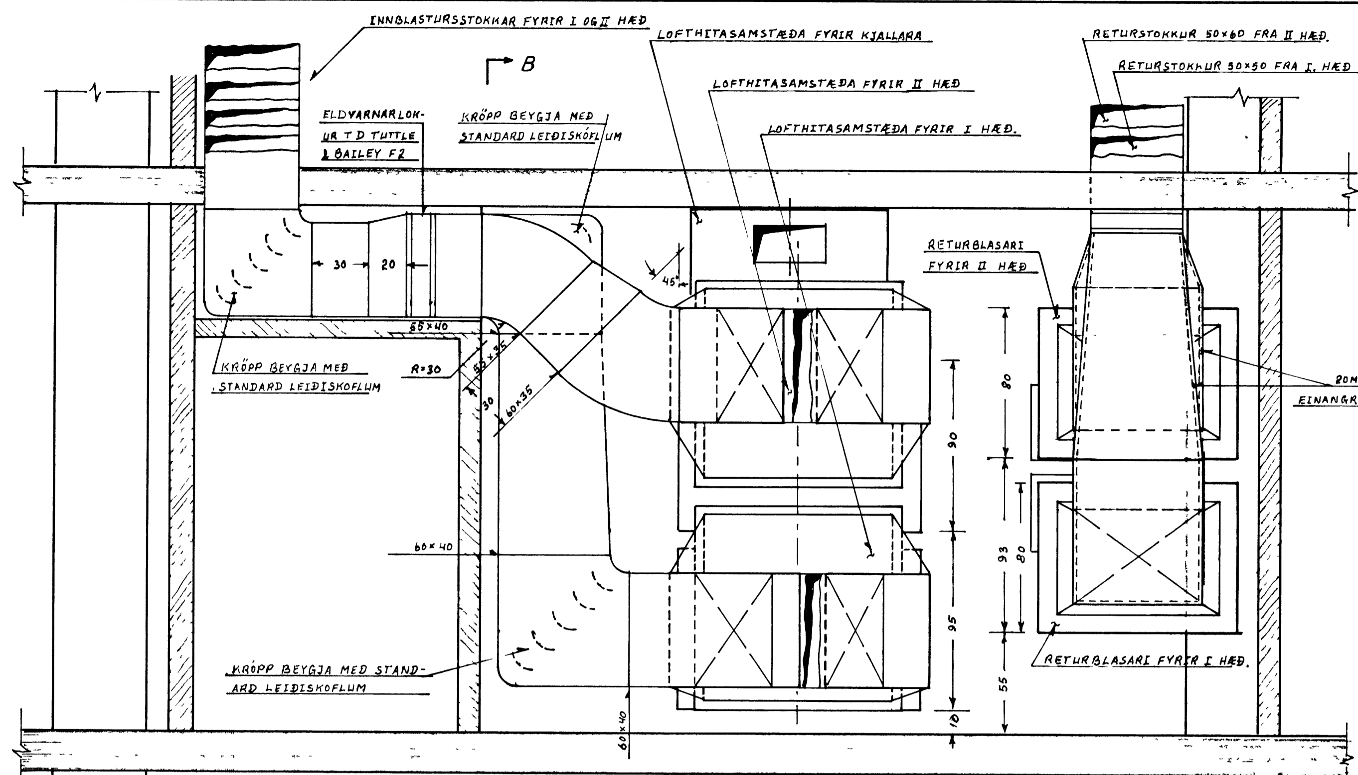
SNEIÐING A-A, 1:20.
