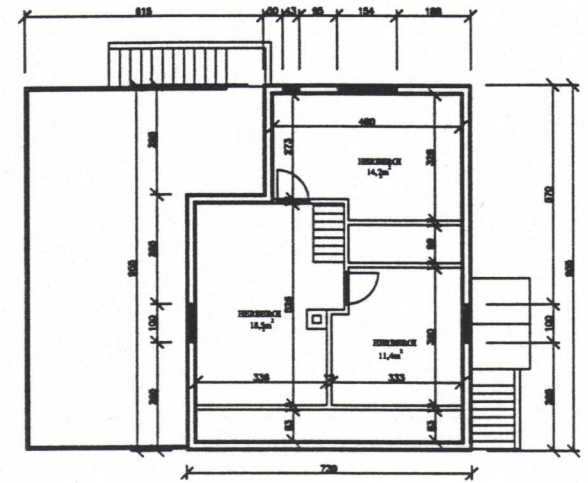
GRUNNMYND RIS M=1:100
