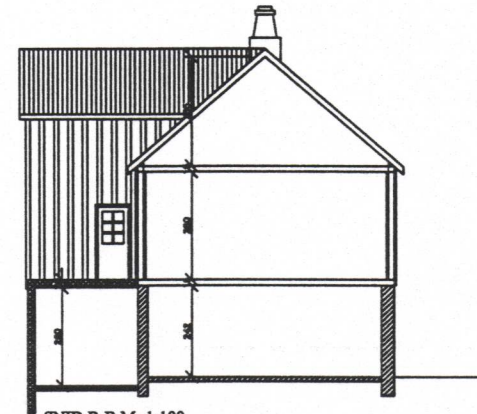
SNIÐ B-B M=1:100
