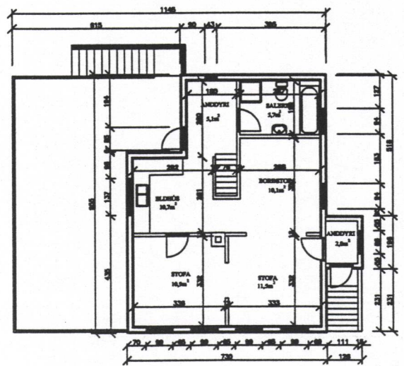
GRUNNMYND 1 HÆÐ M=1:100
