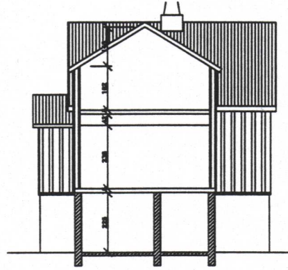
SNIÐ A-A M=1:100
