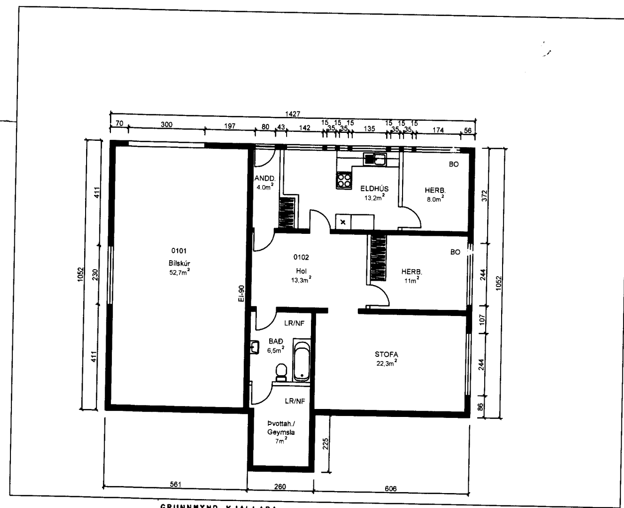
GRUNNMYND KJALLARA
