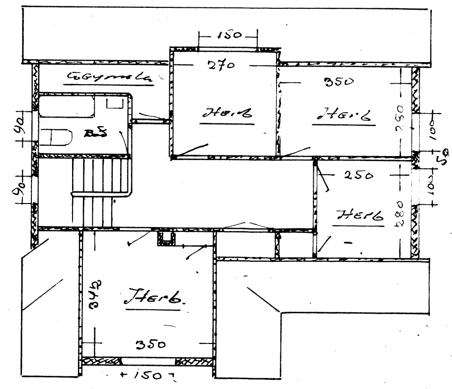
2. HÆÐ 150
