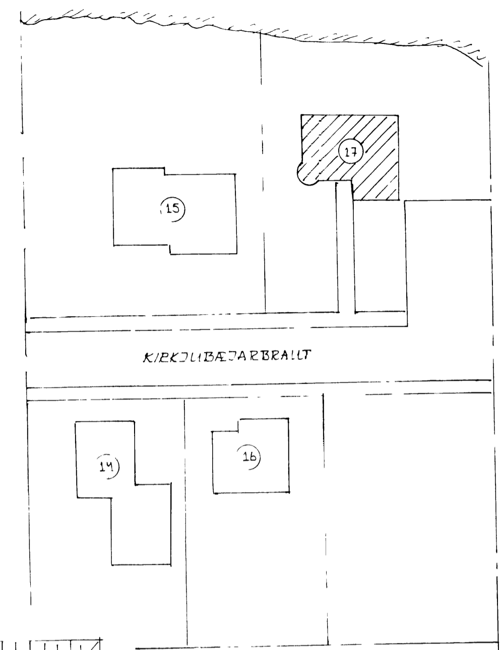
AFSTÖÐUMYND M=1 500
