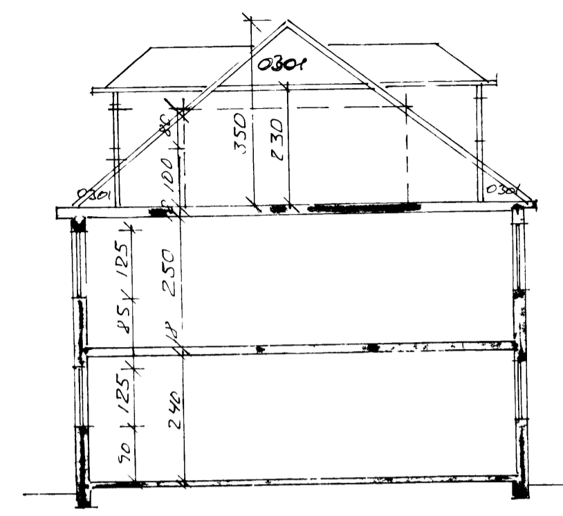
SKURPUR M=1 100
