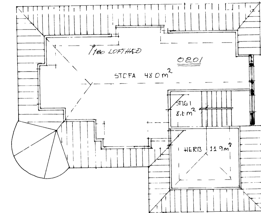
DAGHÆÐ M=1 100
