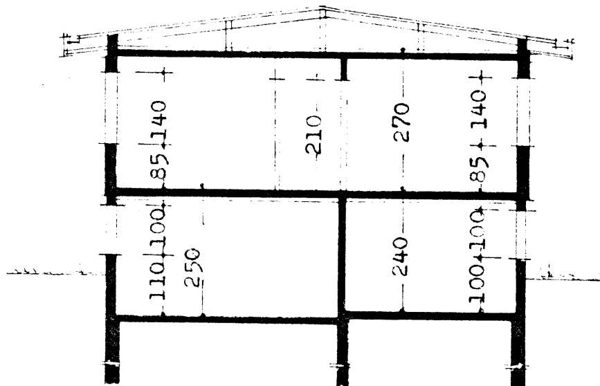
Skurður B-B
