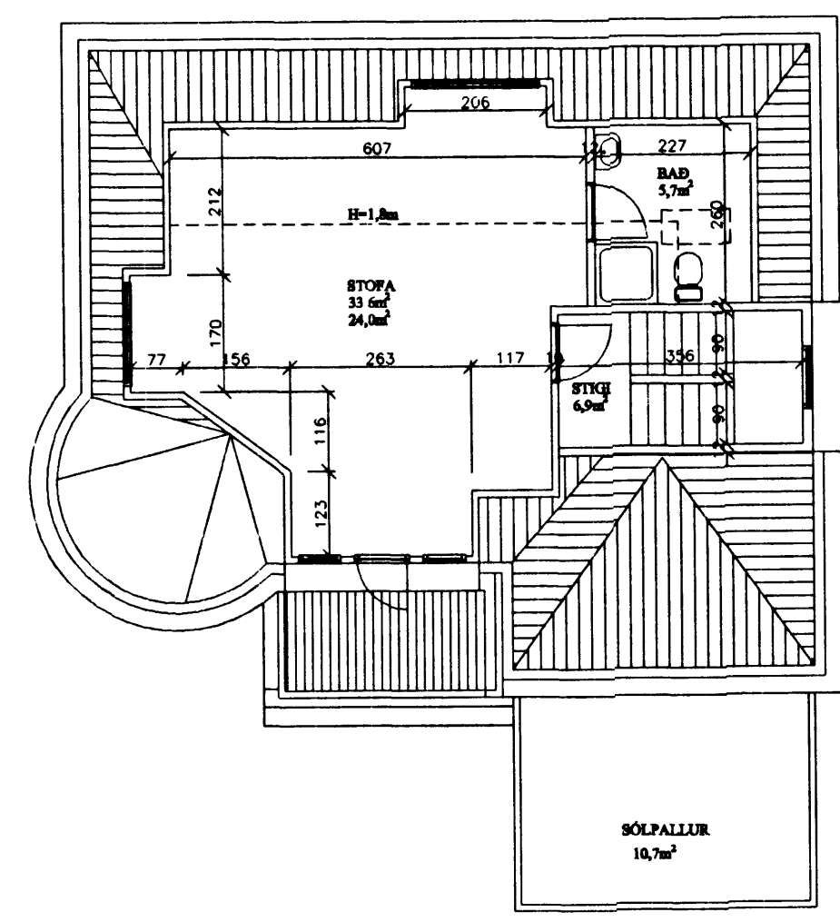
GRUNNMYND 2 HÆÐ M=1:100
