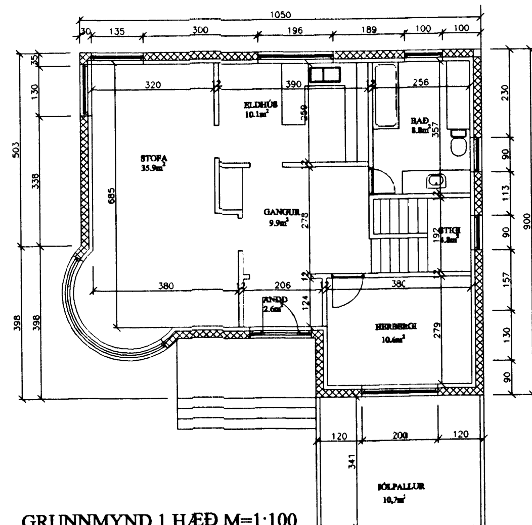
GRUNNMYND 1 HÆÐ M=1:100
