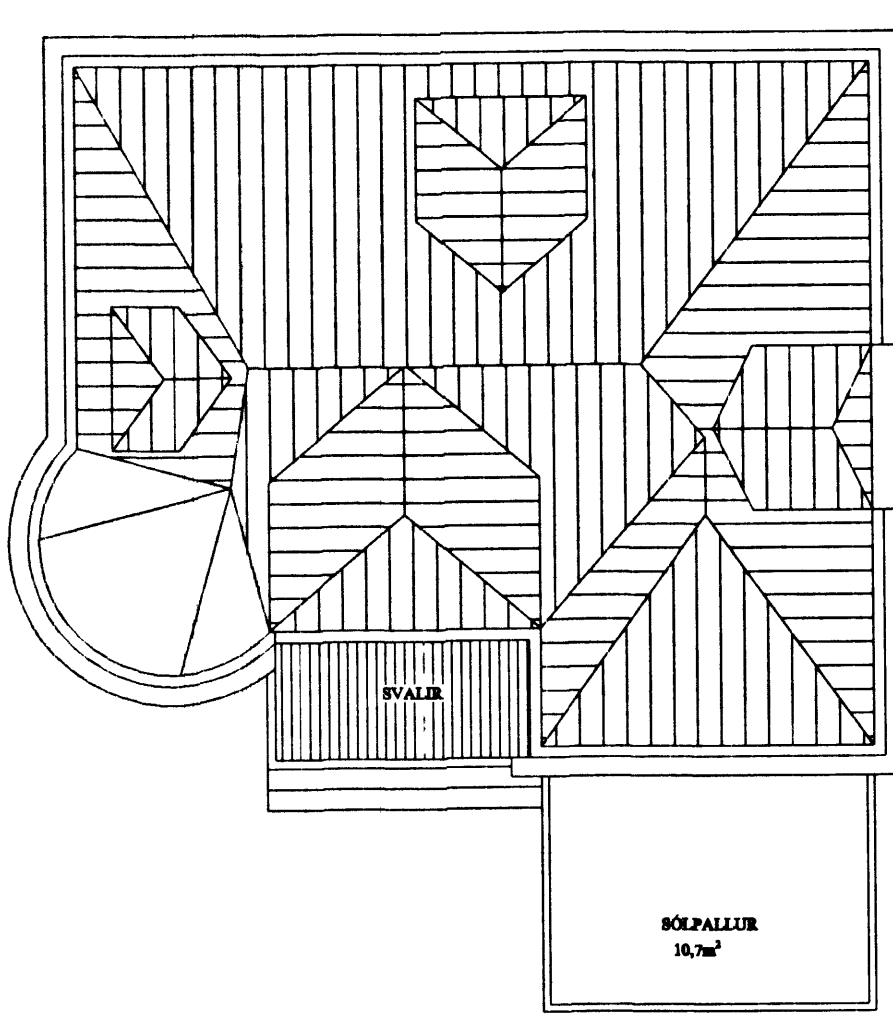
GRUNNMYND ÞAK M=1:100
