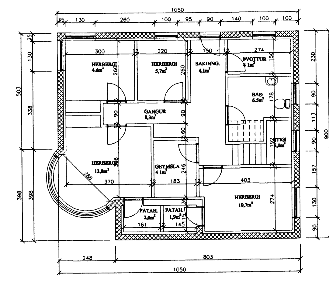
GRUNNMYND KJALLARI M=1:100
