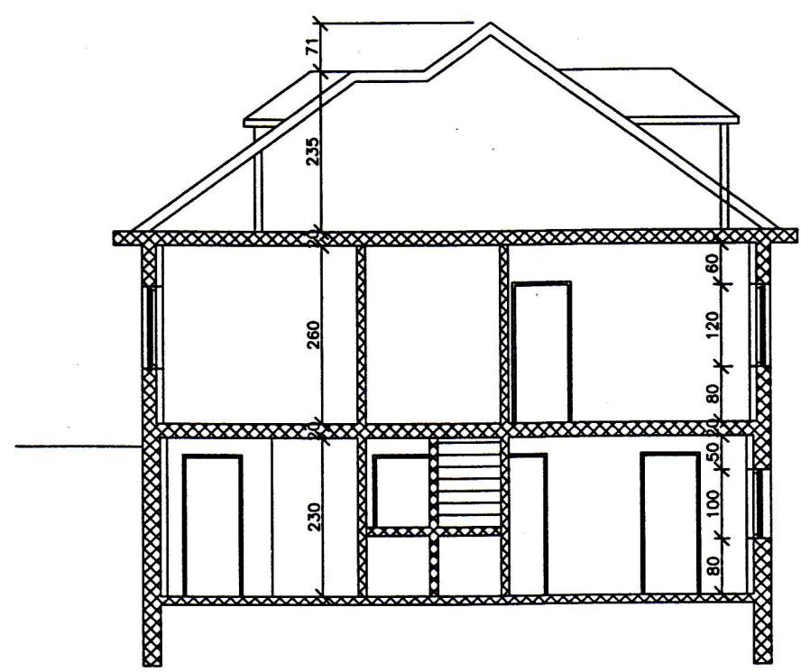
SNIÐ A-A
