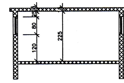
SNIÐ
