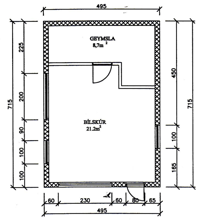
GRUNNMYND BÍLSKÚR
