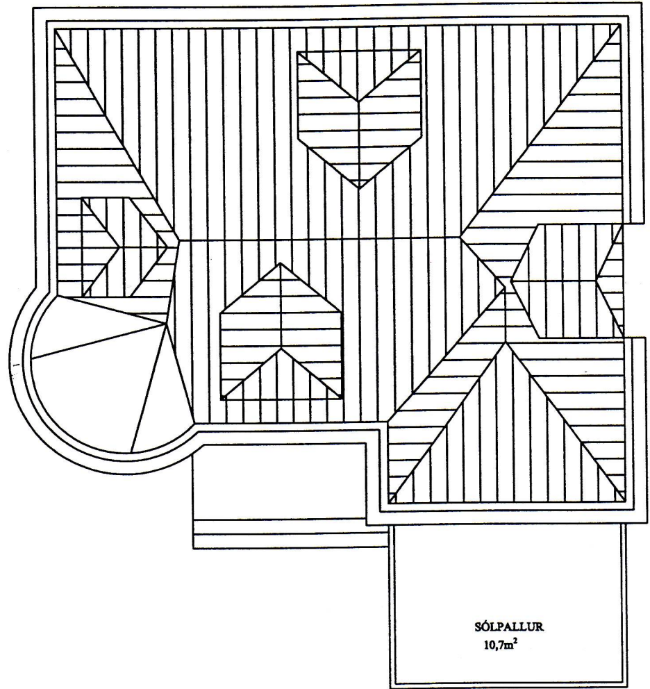
GRUNNMYND ÞAK M=1:100
