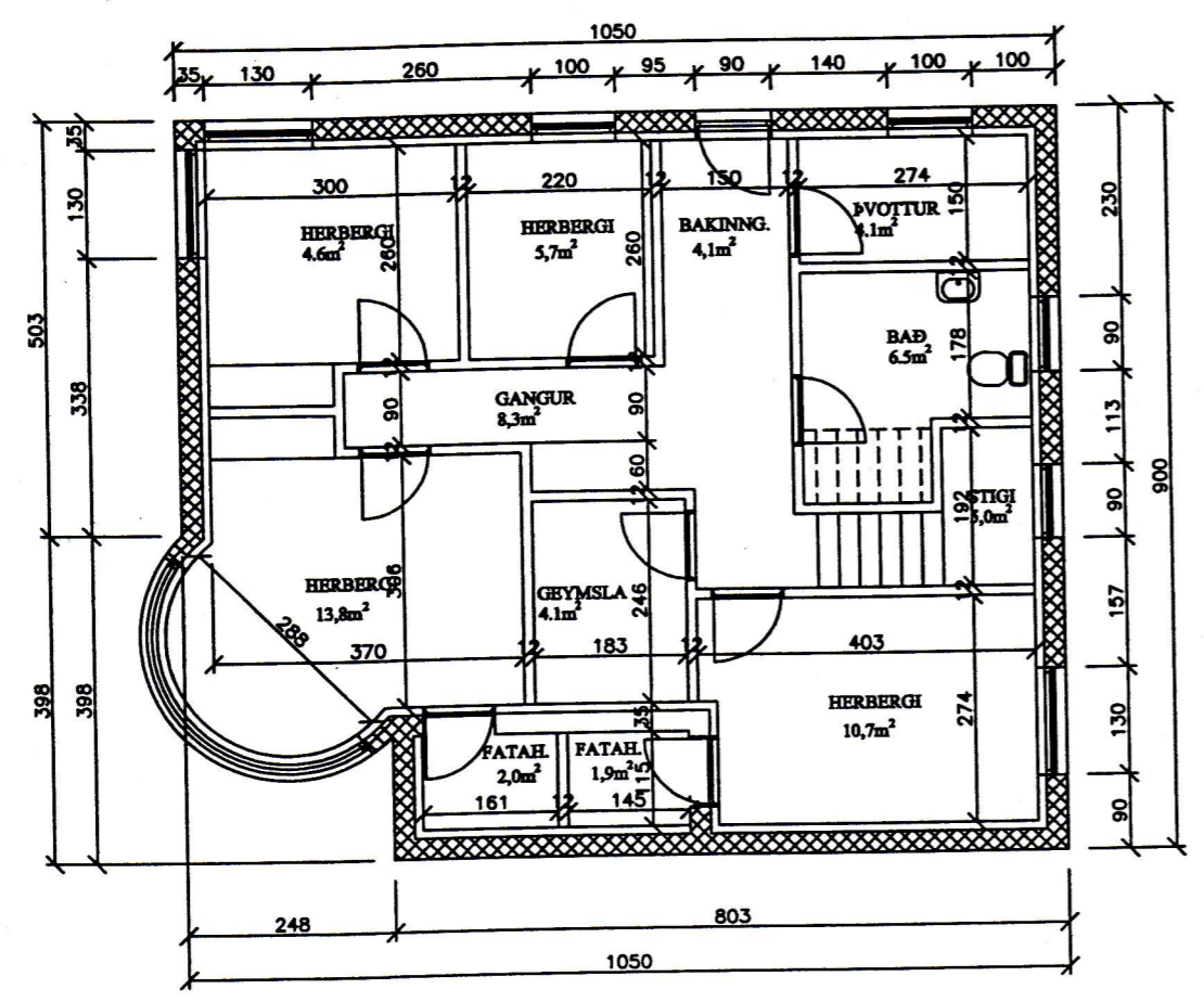
GRUNNMYND KJALLARI M=1:100
